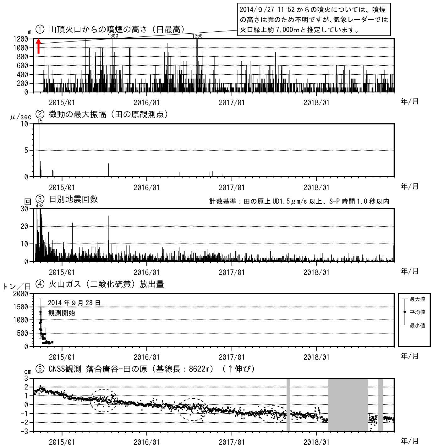
図 3 御嶽山 最近の火山活動経過図（2014 年 9 月 1 日～2018 年 11 月 30 日）
