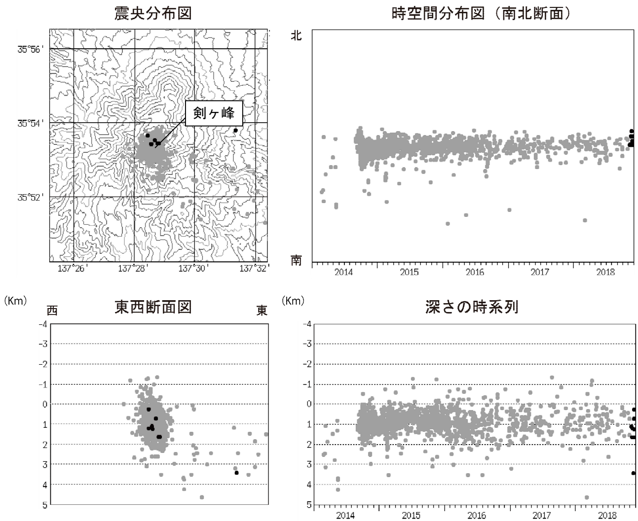
図 5 御嶽山 震源分布図（2014 年 1 月 1 日～2018 年 11 月 30 日）
