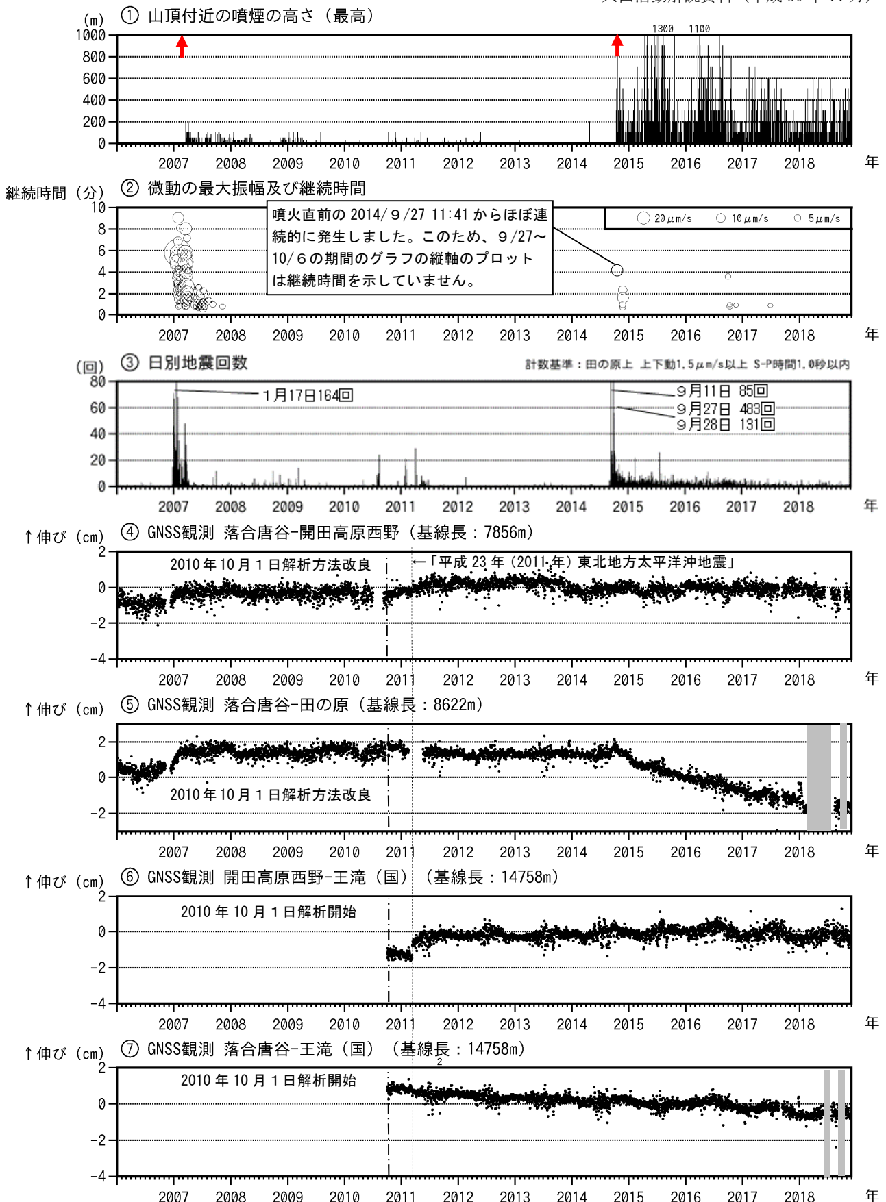
図6 御嶽山 長期間の火山活動経過図（2006年1月1日～2018年11月30日）
