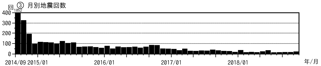
図 4 月別地震回数経過図（2014 年 9 月～2018 年 11 月）
