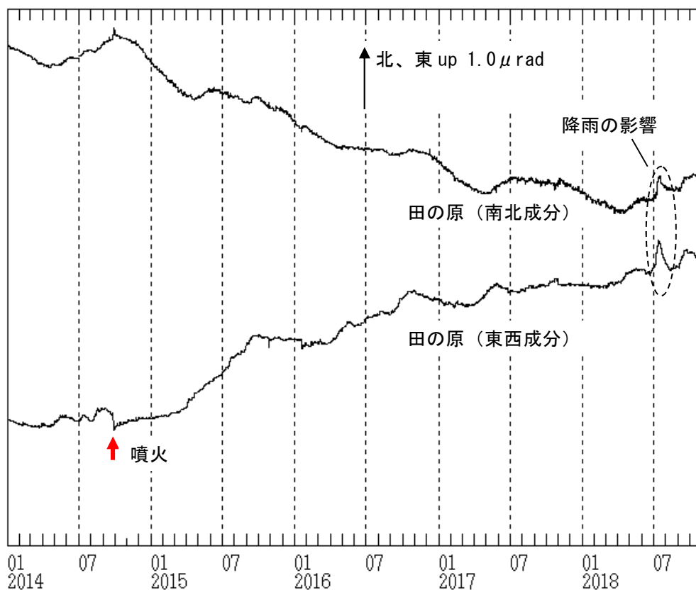
図 8 御嶽山 田の原観測点の傾斜変動（2014 年 1 月 1 日～2018 年 10 月 31 日）
