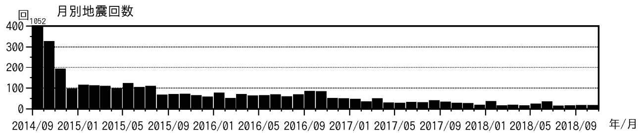
図 4 月別地震回数経過図（2014 年 9 月 1 日～2018 年 10 月 31 日）
