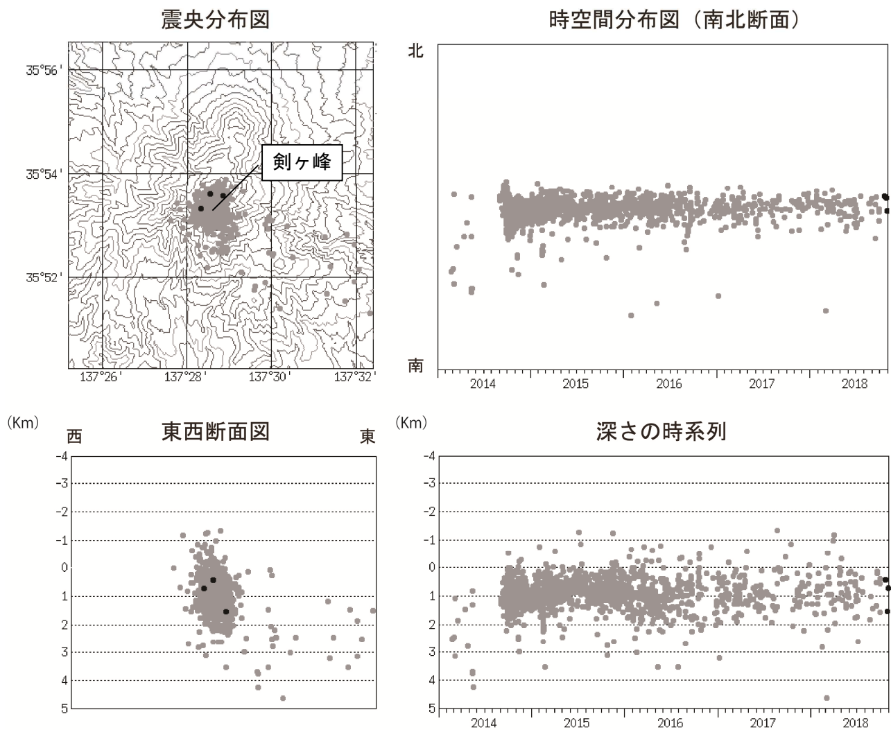
図 5 御嶽山 震源分布図（2014 年 1 月 1 日～2018 年 10 月 31 日）
