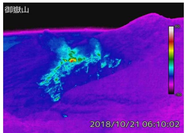
図 2 御嶽山 剣ヶ峰山頂の南西側の火口列の可視画像と地表面温度分布 3) （奥の院監視カメラによる） 3) 赤外熱映像装置により観測しています。赤外熱映像装置は、物体が放射する赤外線を感じて温度を測定する測器で、熱源から離れた場所から測定することができる利点がありますが、測定距離や大気等の影響で実際の温度よりも低く測定される場合があります。
