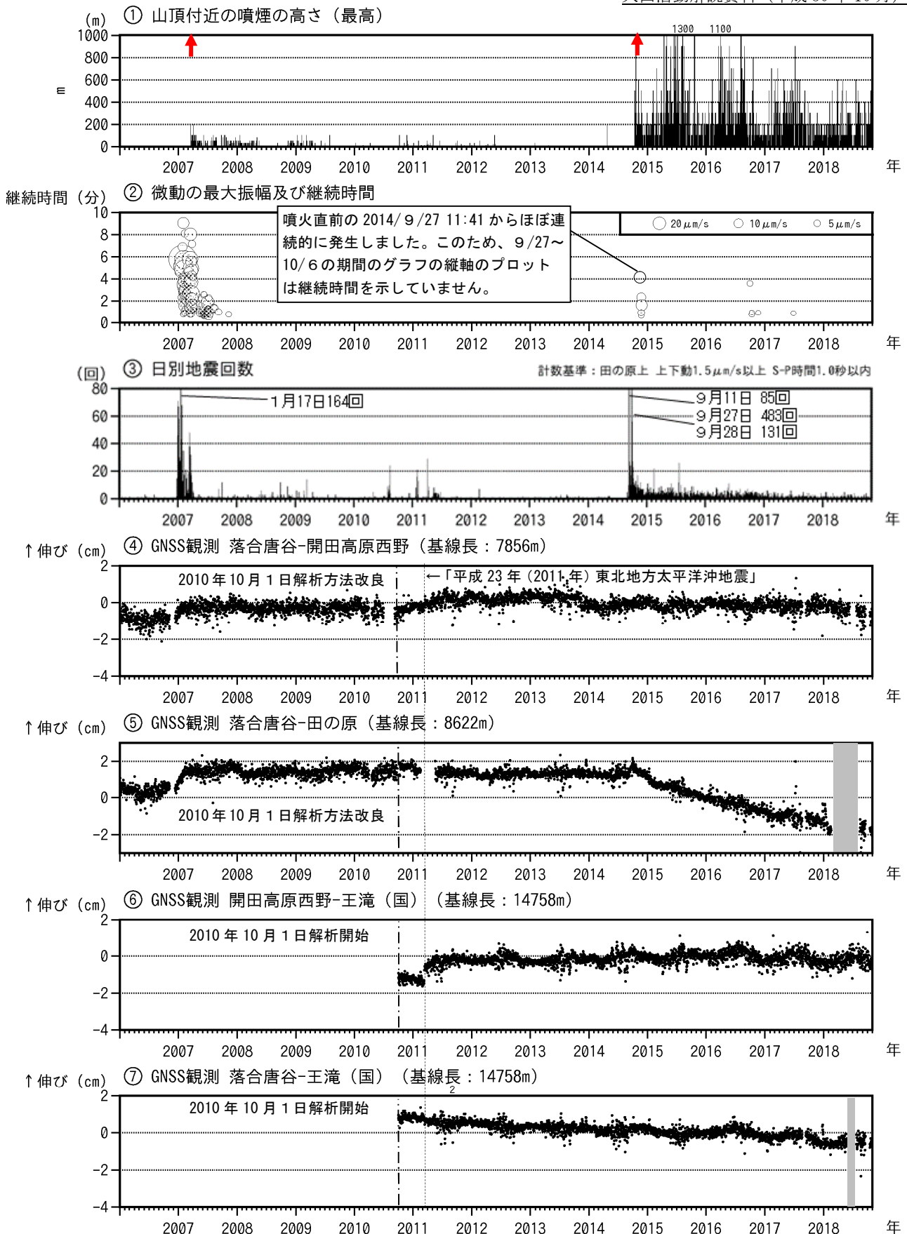
図6 御嶽山 長期間の火山活動経過図（2006年1月1日～2018年10月31日）
