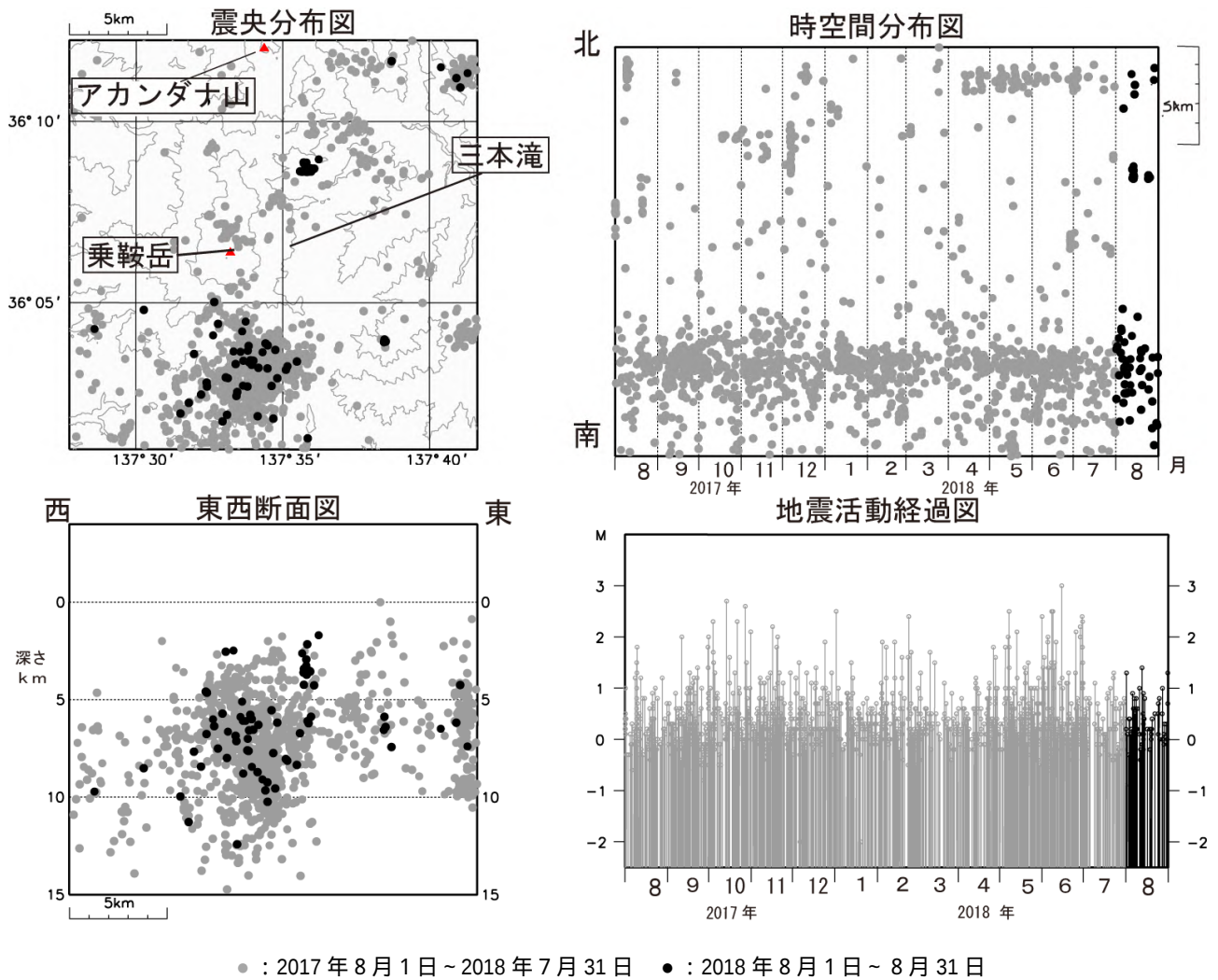
図 3 乗鞍岳 広域地震観測網による山体・周辺の地震活動(2017 年 8 月 1 日 ~ 2018 年 8 月 31 日) 広域地震観測網により震源決定したもので、深さは全て海面以下として決定しています。M (マグニチュード) は地震の規模を表します。図中の震源要素は一部暫定値が含まれており、後日変更することがあります。 ・乗鞍岳付近の地震活動は、低調に経過しています。 ・乗鞍岳から南方へ約 6 km 離れたところでまとまった地震活動がみられますが、構造的な地震で乗鞍岳の火山活動とは関係ないとみています。
