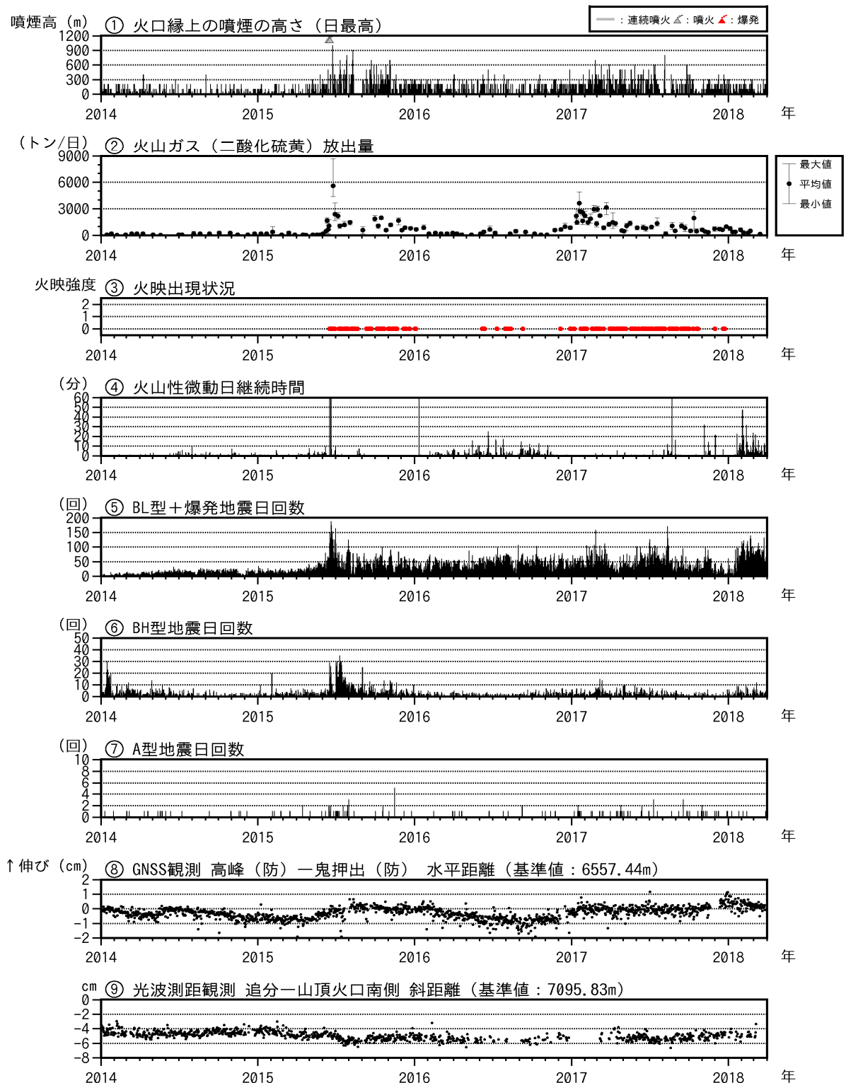
図4 浅間山 最近の火山活動経過図 (2014年1月1日～2018年3月31日)
