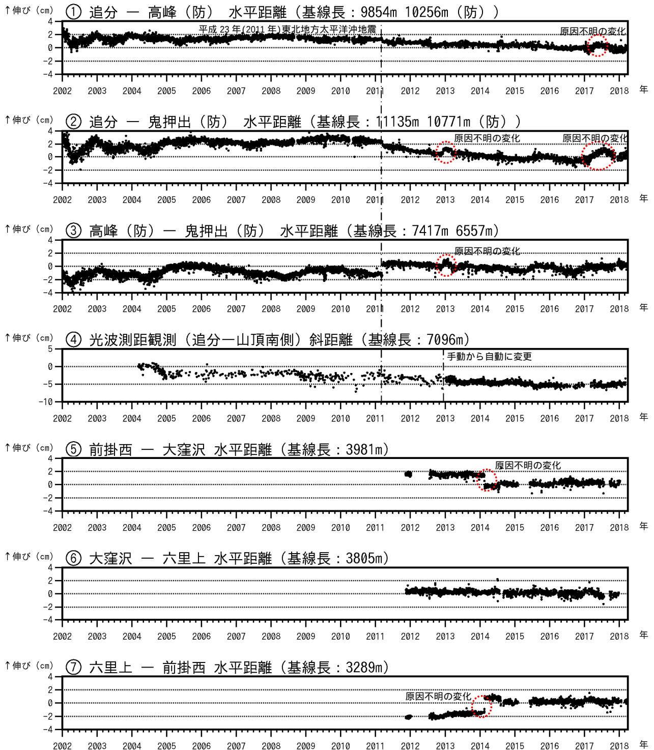
図 6 浅間山 GNSS 連続観測及び光波測距観測の結果(2002 年 1 月 1 日 ~ 2018 年 3 月 31 日)
