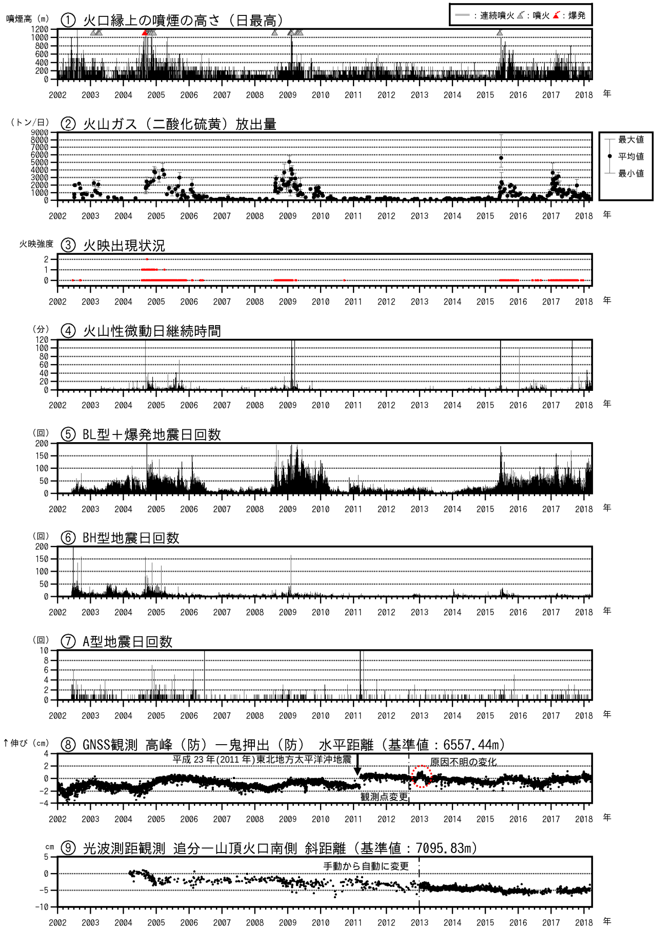
図3 浅間山 火山活動経過図（2002年1月1日～2018年3月31日）
