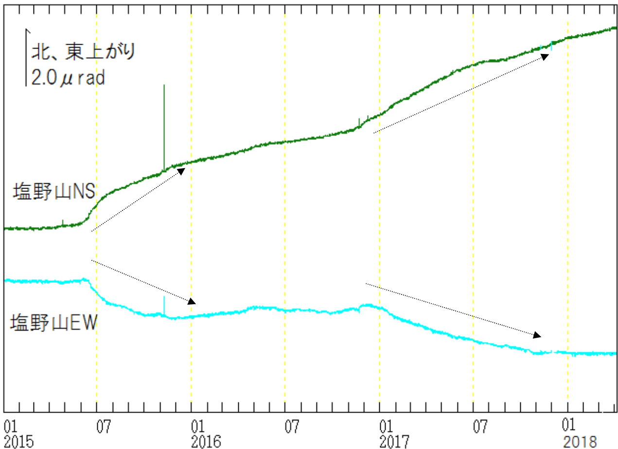
図8 浅間山 塩野山観測点における傾斜データ（2015年1月1日～2018年3月31日）
