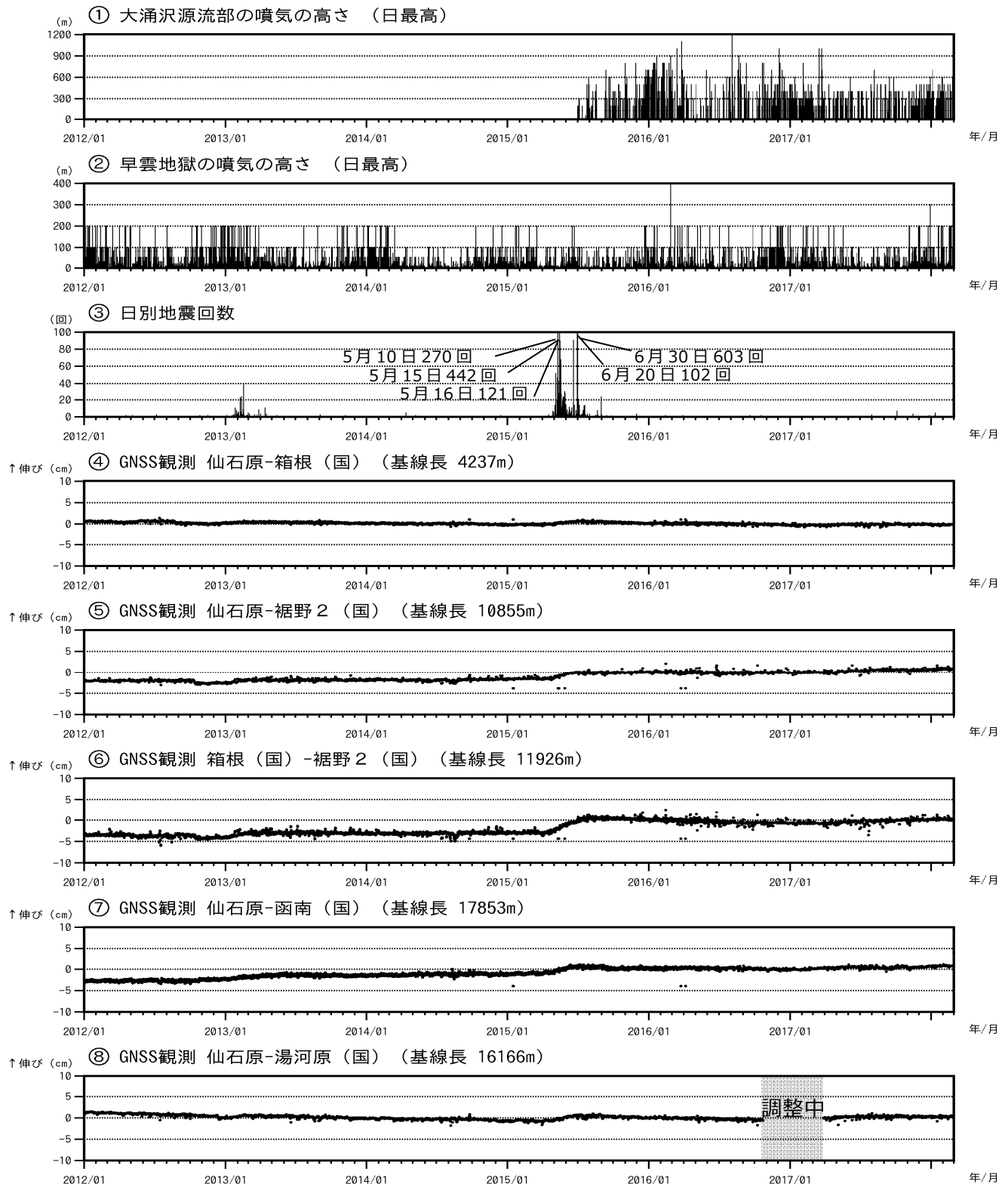
図5 箱根山 火山活動経過図（2012年1月1日～2018年2月28日）
