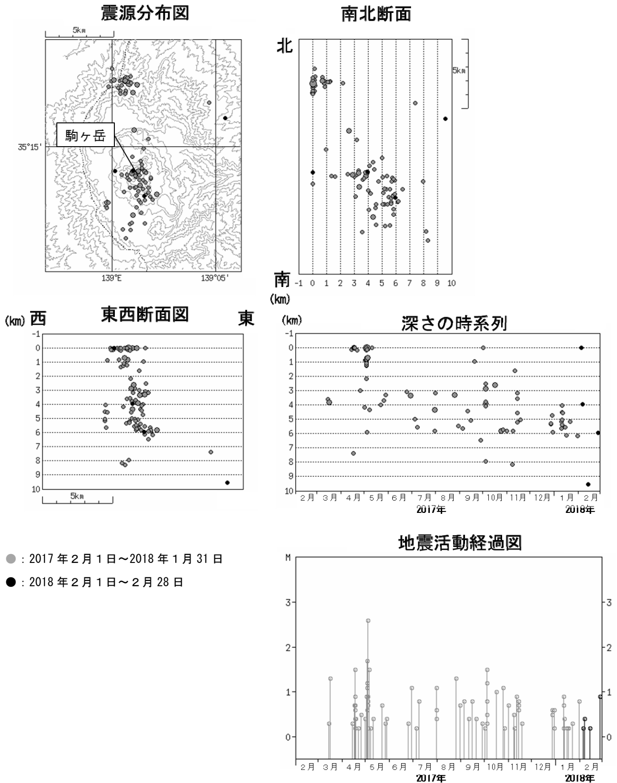
図 6 箱根山 広域地震観測網による山体周辺の震源分布図（2017 年 2 月 1 日～2018 年 2 月 28 日） M（マグニチュード）は地震の規模を表し、M0.2 以上の地震を表示しています。 広域地震観測網により震源決定したもので、深さは全て海面以下として決定しています。 図中の震源要素は一部暫定値が含まれており、後日変更することがあります。
