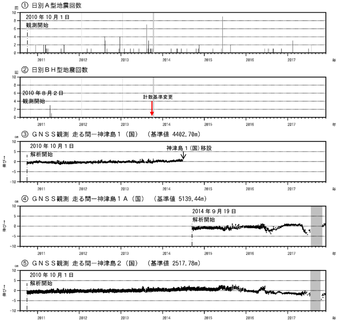
図 3 神津島 火山活動経過図(2010 年 8 月 2 日～2017 年 11 月 30 日)
