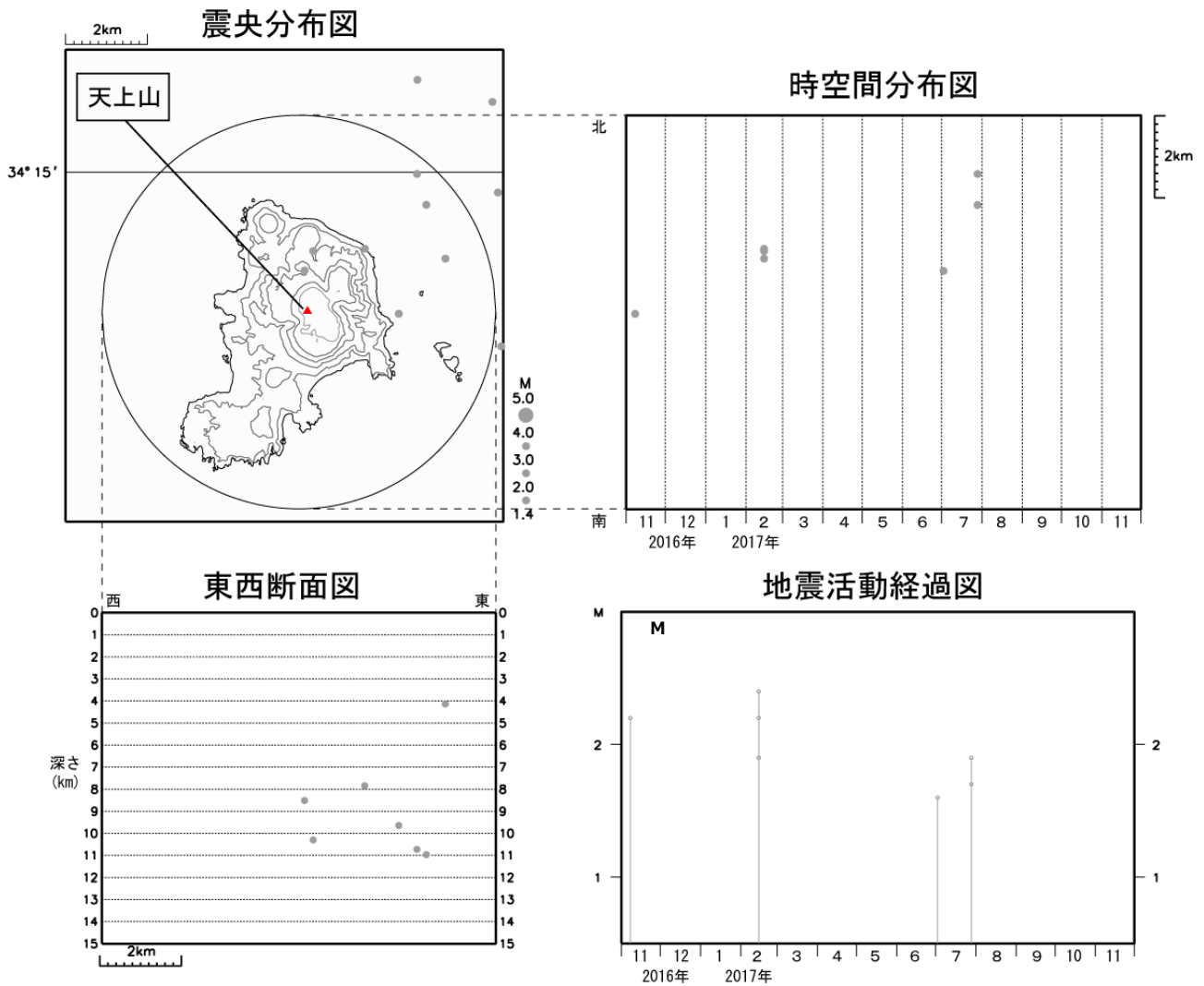
図 4 神津島 広域地震観測網による山体・周辺の地震活動（2016 年 11 月 1 日～2017 年 11 月 30 日）
