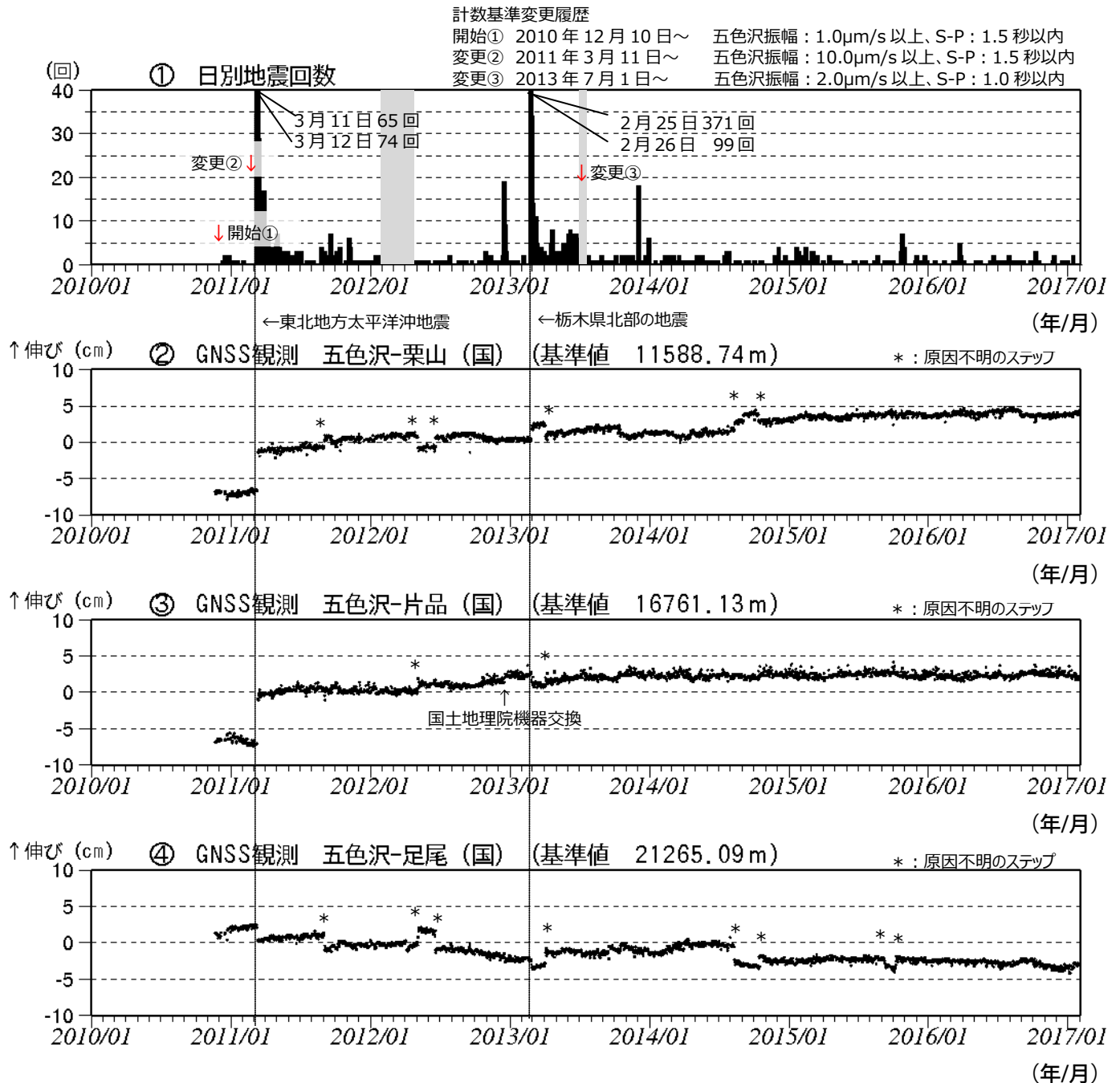
図2 日光白根山 火山活動経過図（2010 年 11 月 20 日～2017 年 1 月 31 日）
