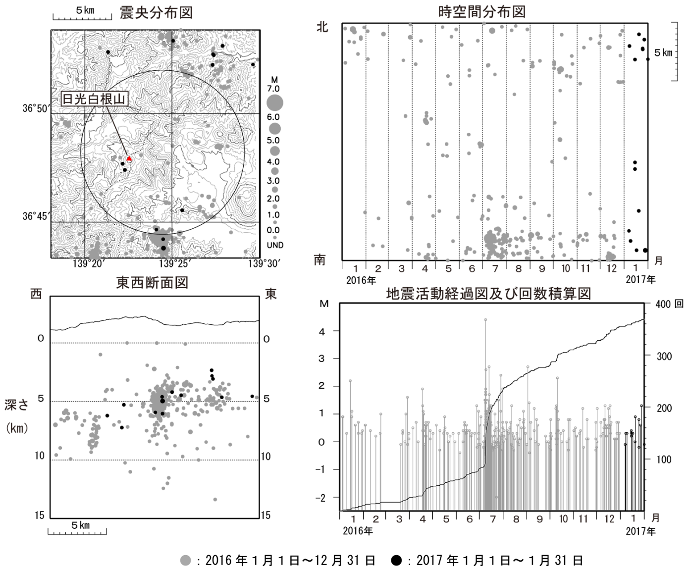
図3 日光白根山 広域地震観測網による山体・周辺の地震活動(2016年1月1日～2017年1月31日)
