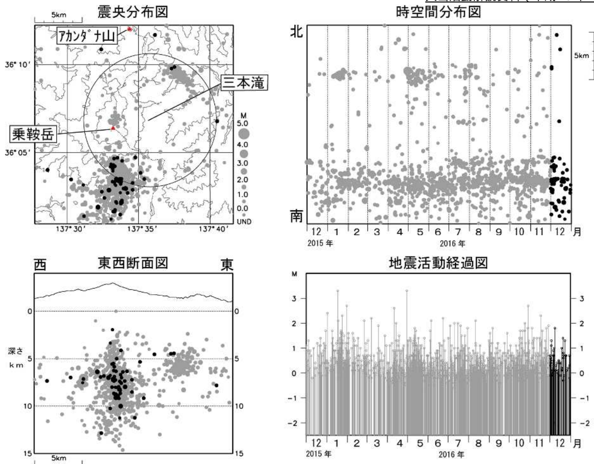
図 3 乗鞍岳 広域地震観測網による山体・周辺の地震活動(2015 年 12 月 1 日～2016 年 12 月 31 日) ● : 2015 年 12 月 1 日～2016 年 11 月 30 日 ● : 2016 年 12 月 1 日～12 月 31 日 ・震央分布図中の円は図 2 - の計数対象地震（三本滝で S - P 時間 1 秒以内）のおよその範囲を示しています。 ・M（マグニチュード）は地震の規模を表します。 ・図中の震源要素は一部暫定値が含まれており、後日変更することがあります。
