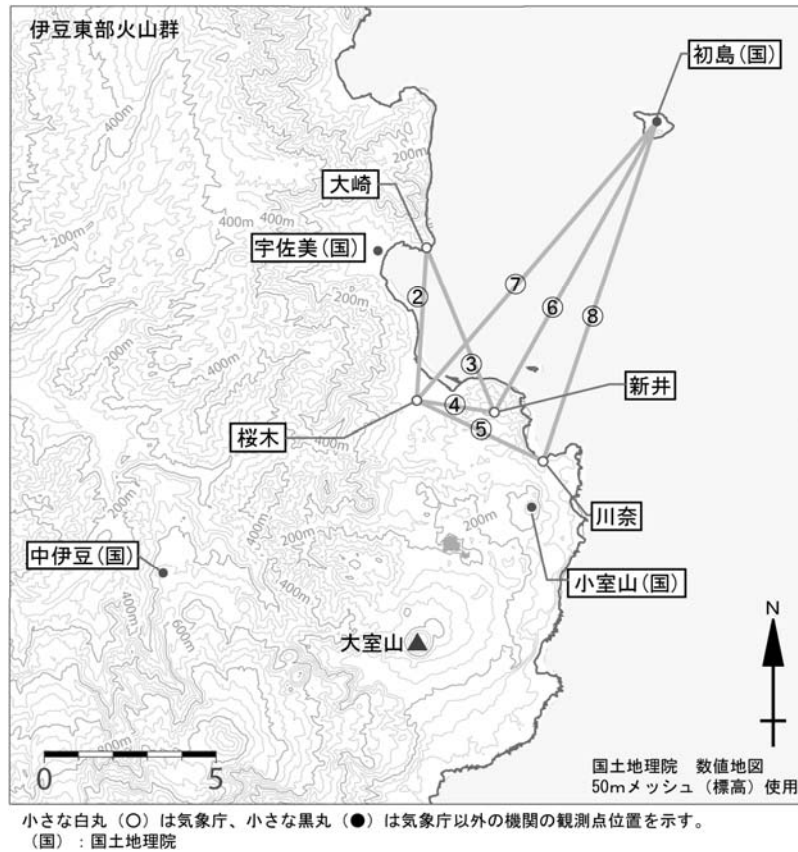
図4 伊豆東部火山群 GNSS 連続観測点配置図
