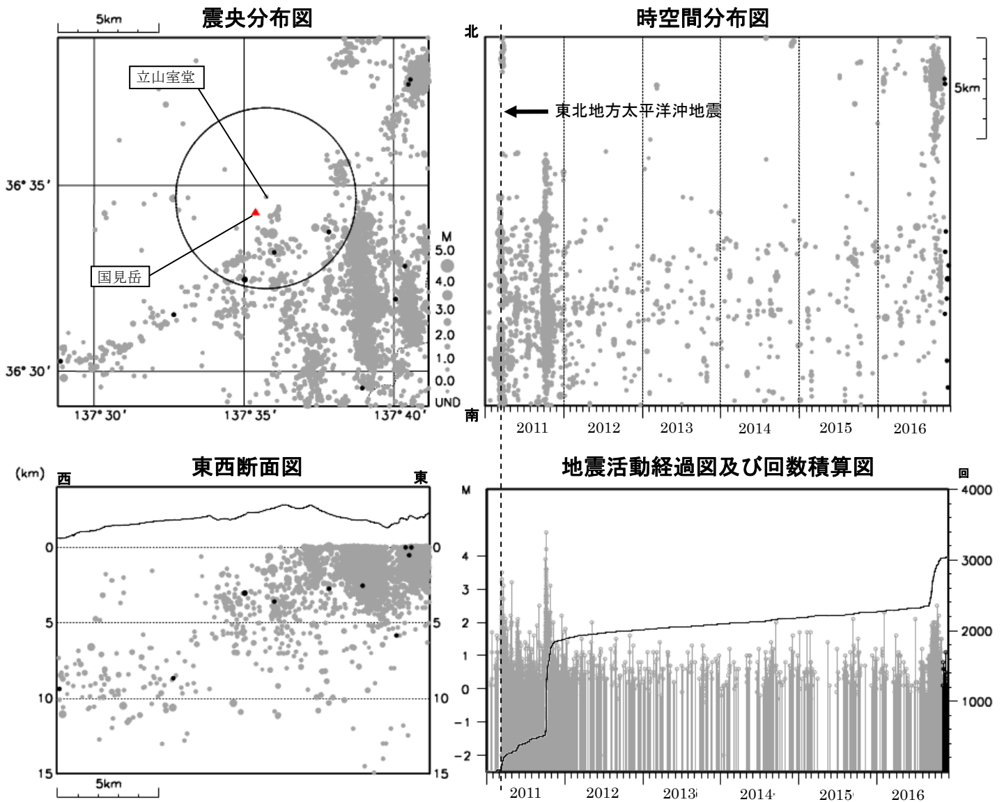
図2 弥陀ヶ原 広域地震観測網による山体・周辺の地震活動（2011年1月1日～2016年11月30日）
