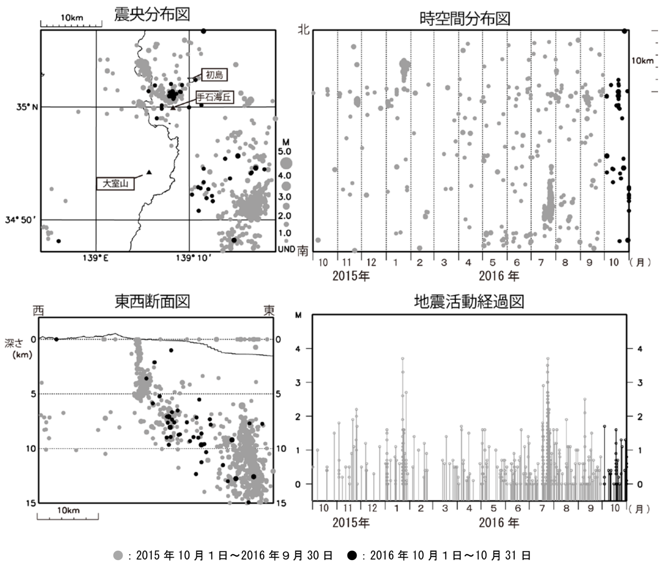
図 2 伊豆東部火山群 広域地震観測網による震源分布図（2015 年 10 月 1 日～2016 年 10 月 31 日）
