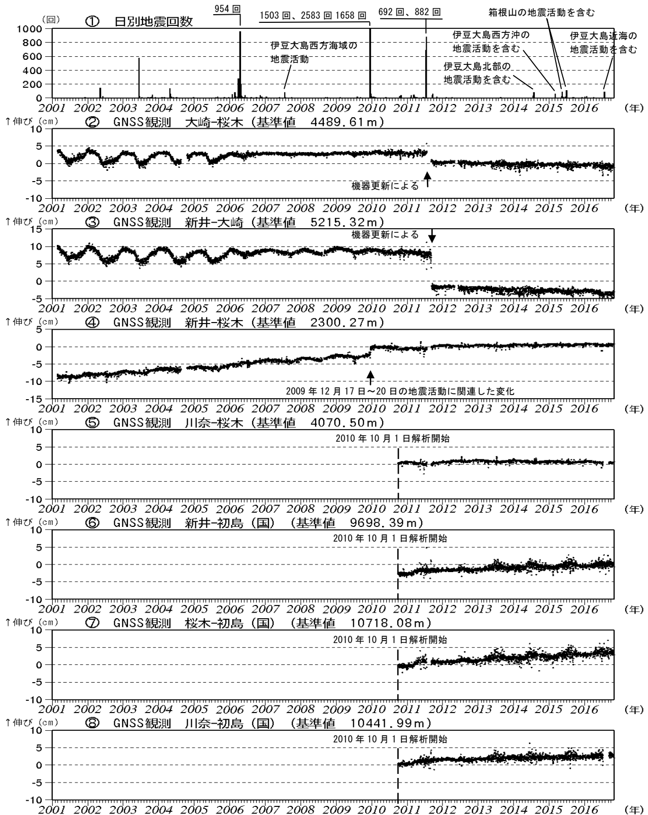
図3 伊豆東部火山群 火山活動経過図（2001年1月1日～2016年10月31日）
