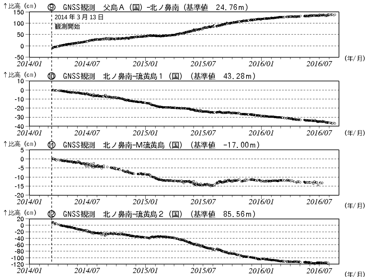
図7 硫黄島 GNSS 観測結果（2014年3月13日～2016年8月31日）（国）：国土地理院
