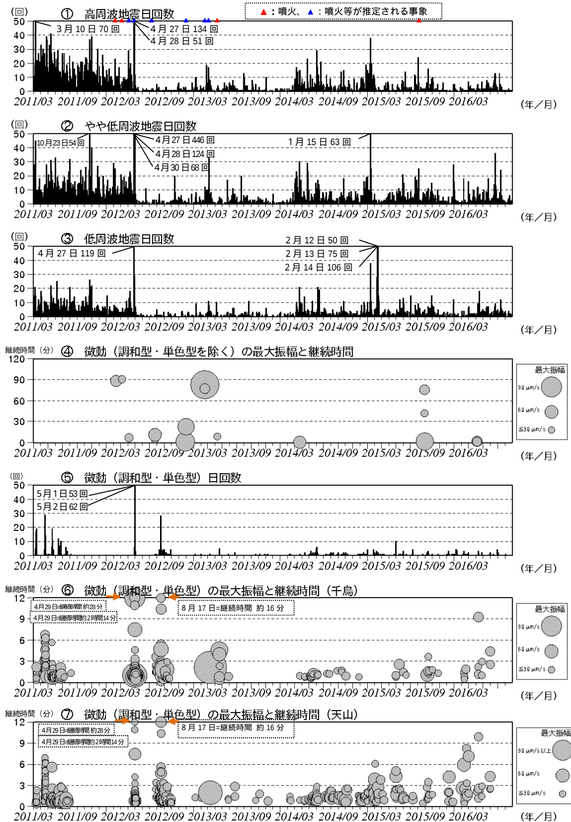
図5 硫黄島 火山活動経過図（2011年3月8日～2016年8月31日）
