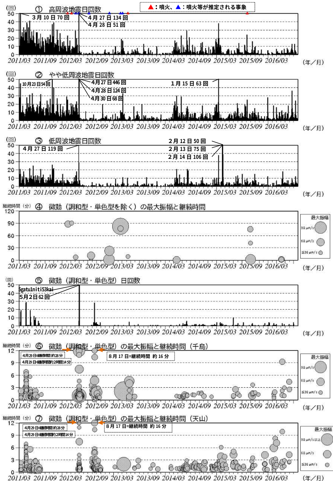
図5 硫黄島 火山活動経過図（2011年3月8日～2016年7月31日）
