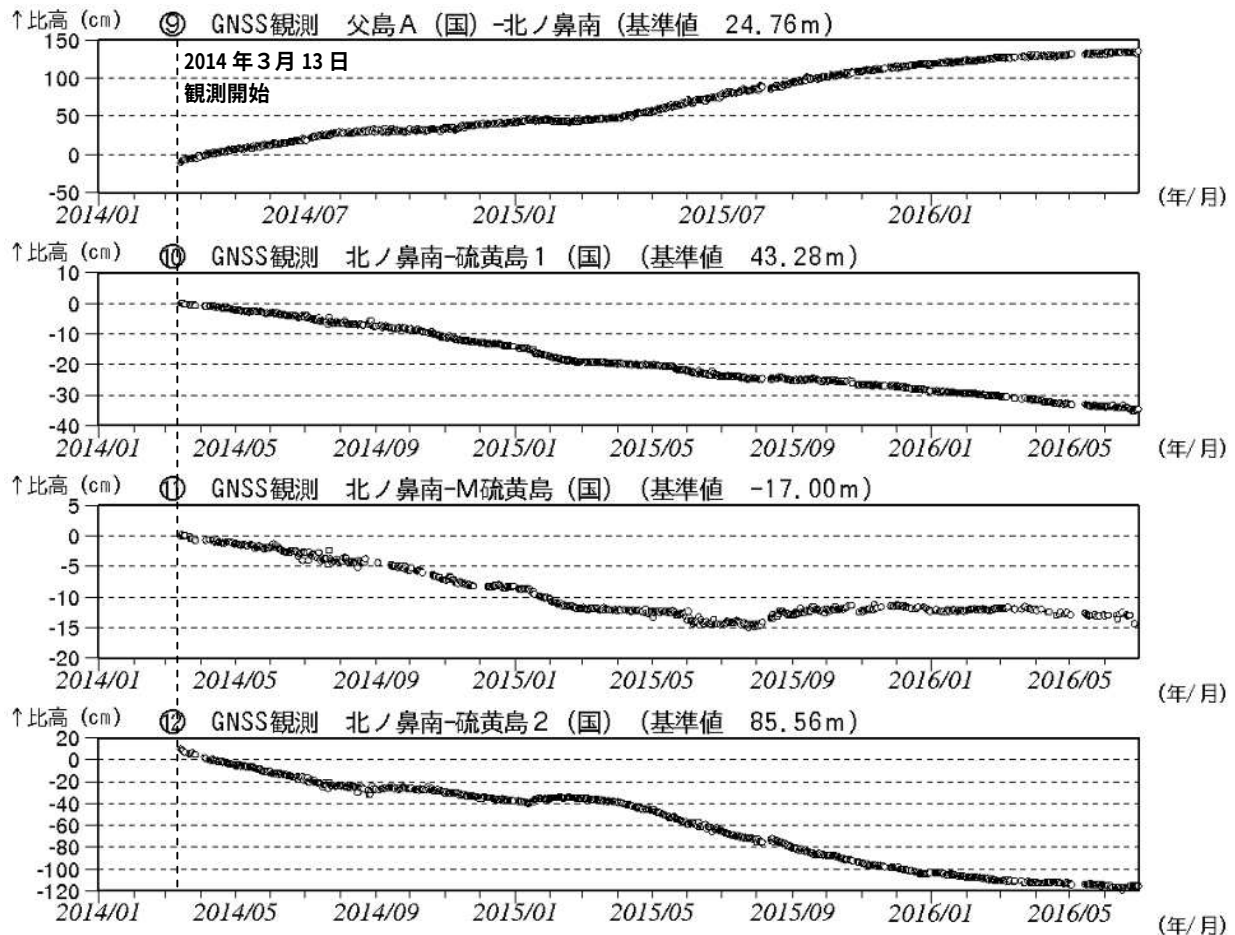
図7 硫黄島 GNSS 1) 観測結果 (2014年3月13日～2016年7月31日) (国): 国土地理院 ・ 基線⑨～⑫は図8の⑨～⑫に対応します。いずれの図も、左の観測点に対する右の観測点の比高（高度の差）の変化を表しています。グラフの空白部分は欠測を示します。 ・ 北ノ鼻南観測点は2014年3月13日から観測を開始しました。
