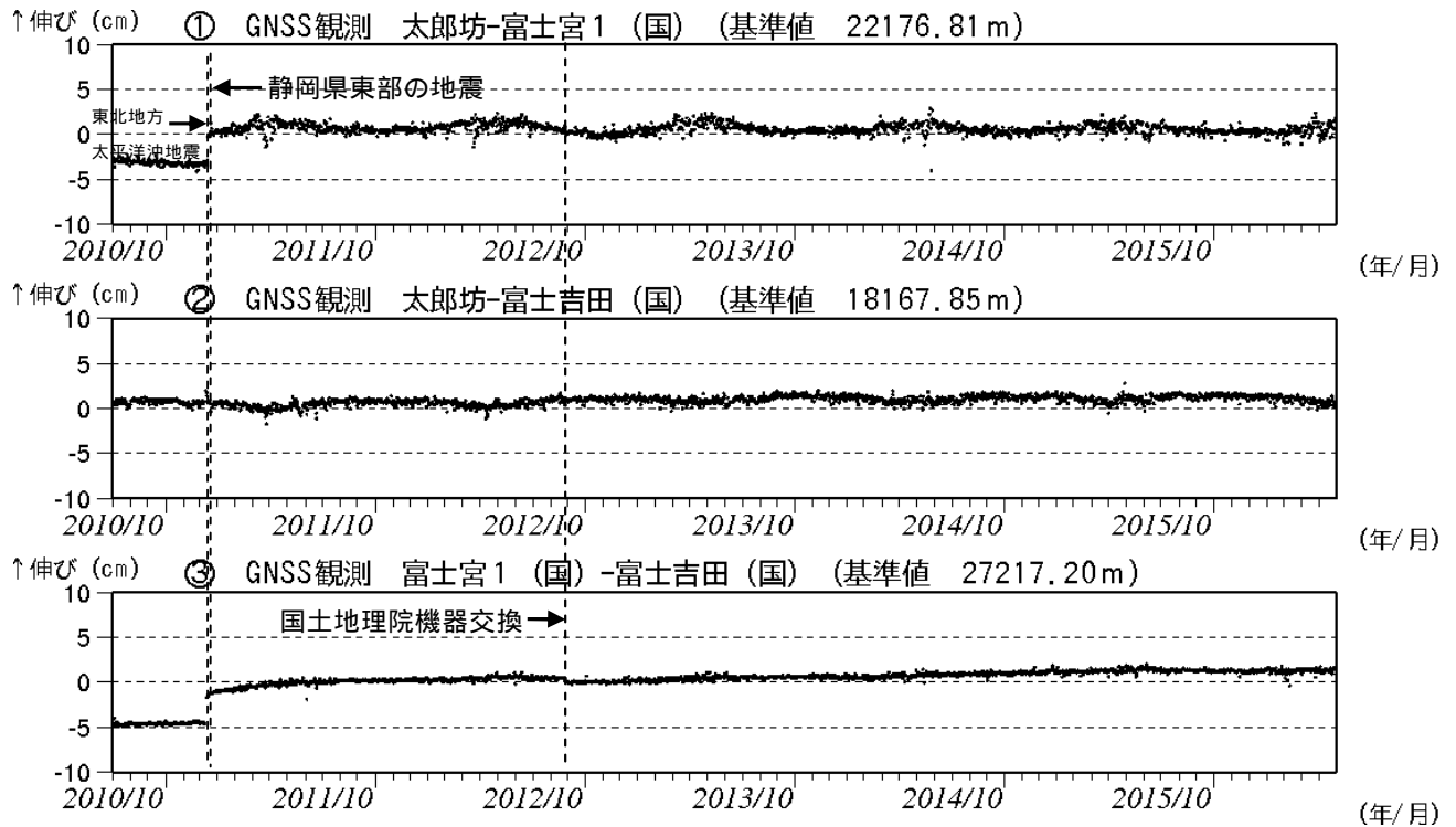
図4 富士山 GNSS 連続観測による基線長変化（2010 年 10 月 1 日～2016 年 7 月 31 日） （国）：国土地理院
