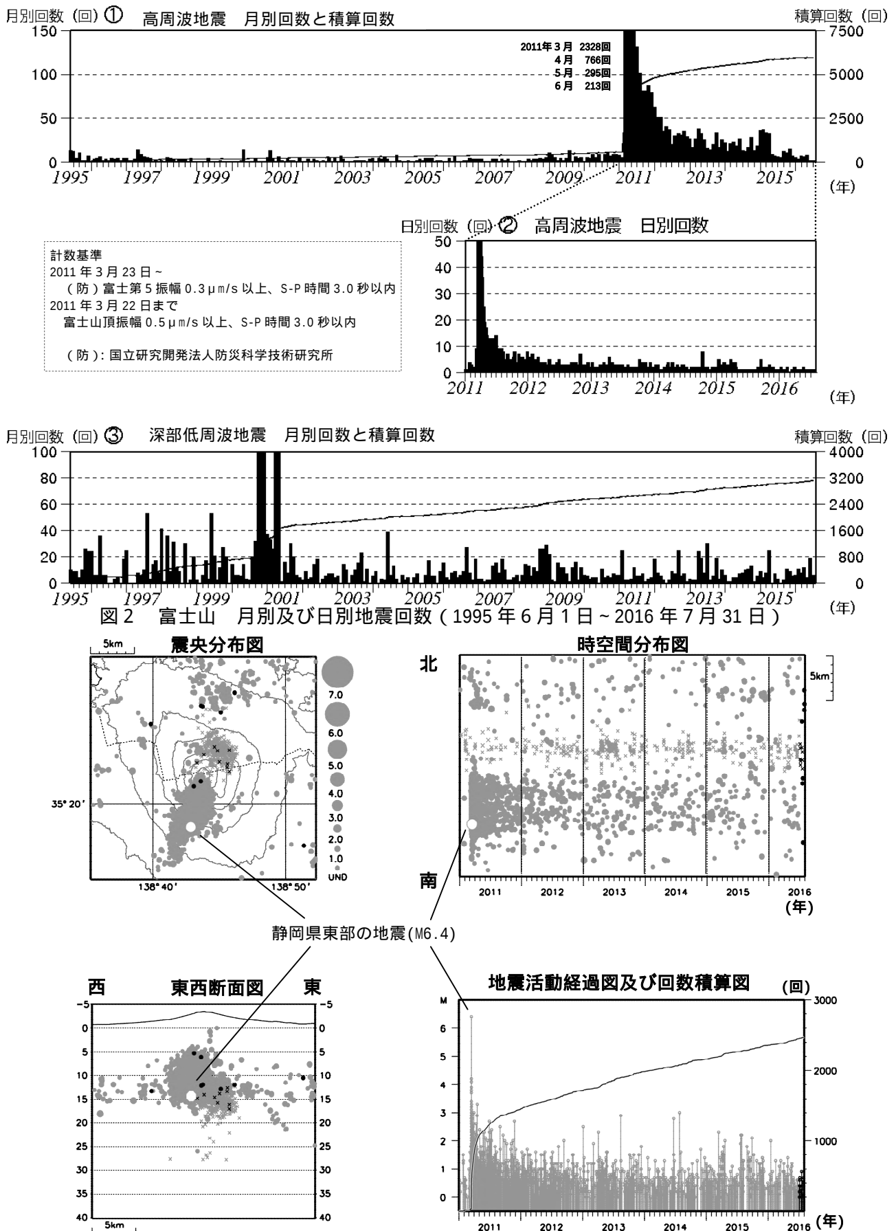
図 3 富士山 広域地震観測網による山体・周辺の地震活動（2011 年 1 月 1 日～2016 年 7 月 31 日）
