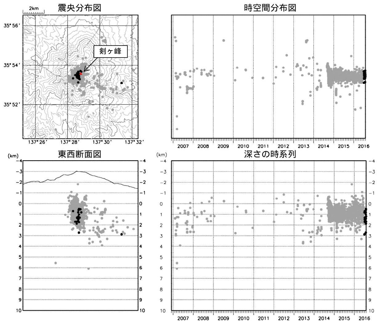
図 2 御嶽山 震源分布図（2006 年 12 月 1 日～2016 年 7 月 31 日）
