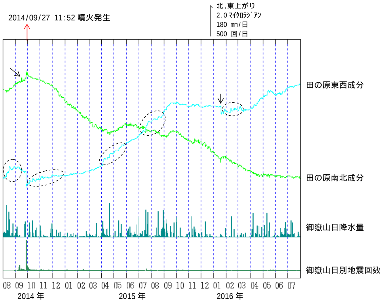
図5 御嶽山 田の原観測点（剣ヶ峰山頂の南東約3 km）の傾斜変動 （2014年8月1日～2016年7月31日）
