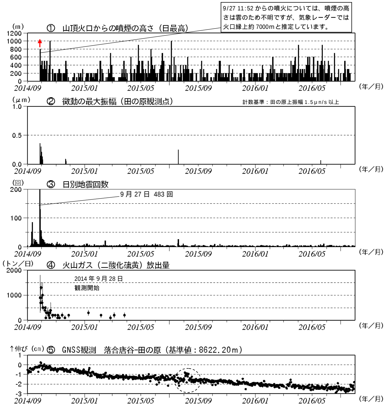
図3 御嶽山 最近の火山活動経過図（2014 年 9 月 1 日～2016 年 7 月 31 日）
