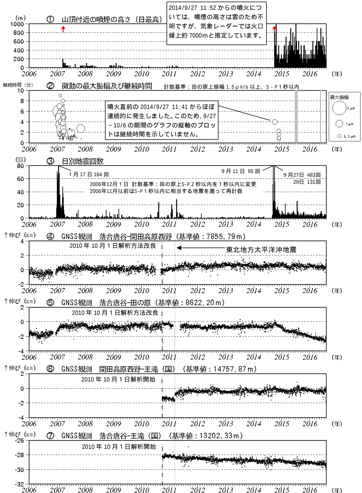
図 4 御嶽山 長期間の火山活動経過図（2006 年 1 月 1 日～2016 年 7 月 31 日）
