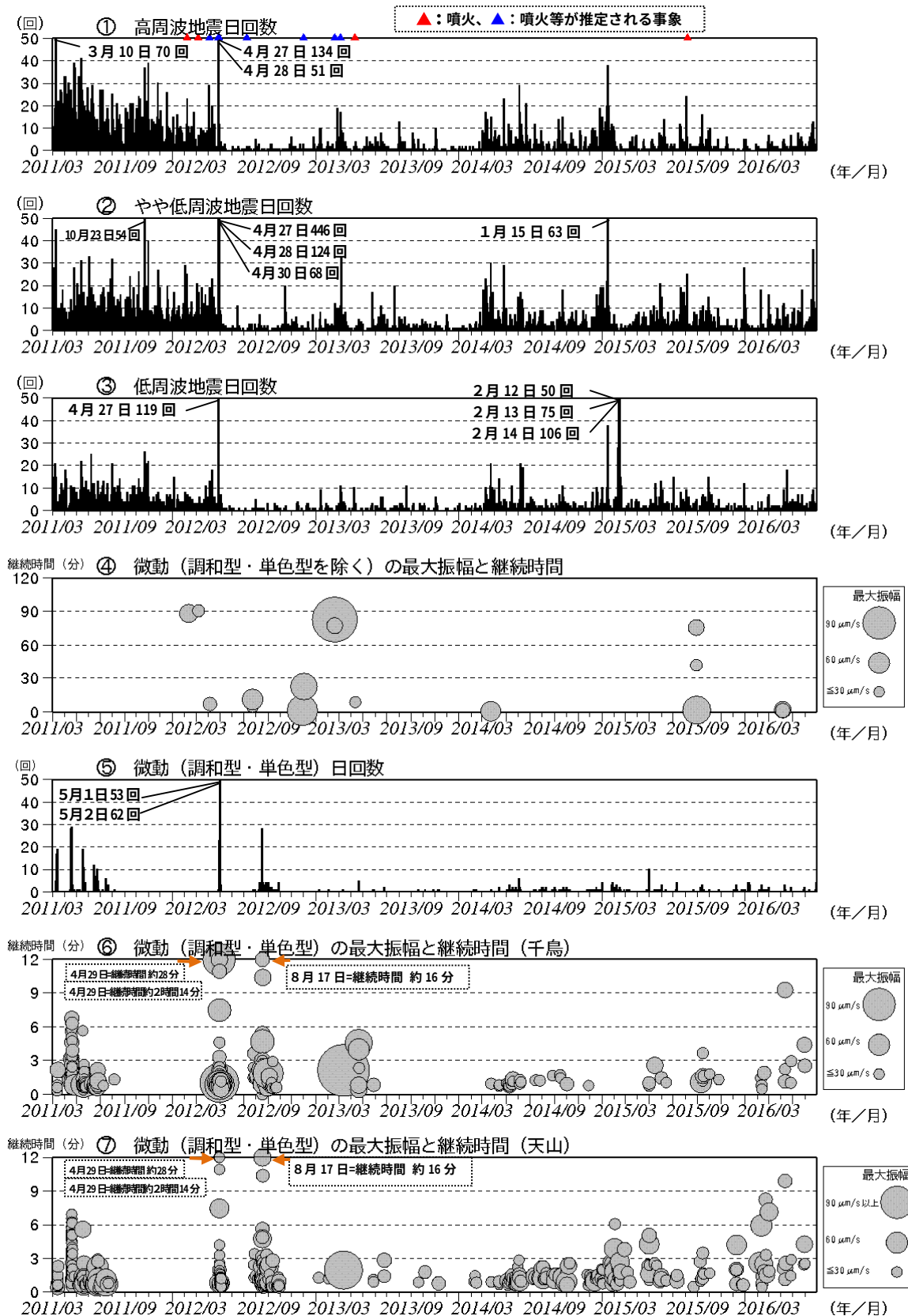
図5 硫黄島 火山活動経過図（2011年3月8日～2016年6月30日）
