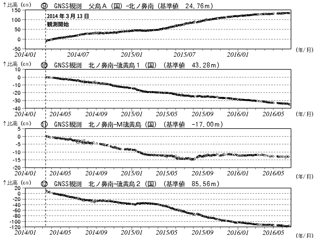
図7 硫黄島 GNSS 1) 観測結果 (2014年3月13日～2016年6月30日) (国)：国土地理院 ・基線⑨～⑫は図8の⑨～⑫に対応します。いずれの図も、左の観測点に対する右の観測点の比高（高度の差）の変化を表しています。グラフの空白部分は欠測を示します。 ・北ノ鼻南観測点は2014年3月13日から観測を開始しました。 ・2014年以降は島の北部ほど隆起が大きい状態が継続しています。
