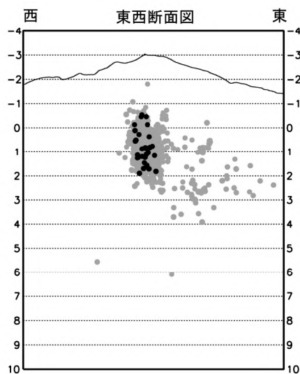
図 2 御嶽山 震源分布図（2006 年 12 月 1 日～2016 年 6 月 30 日）
