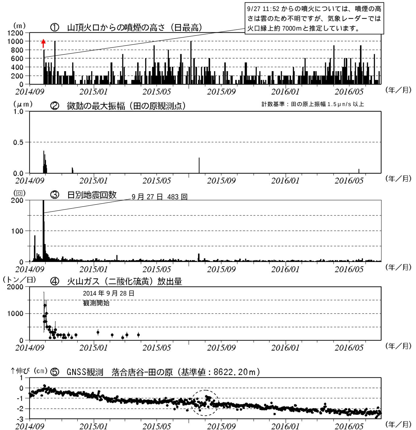
図3 御嶽山 最近の火山活動経過図（2014 年 9 月 1 日～2016 年 6 月 30 日）
