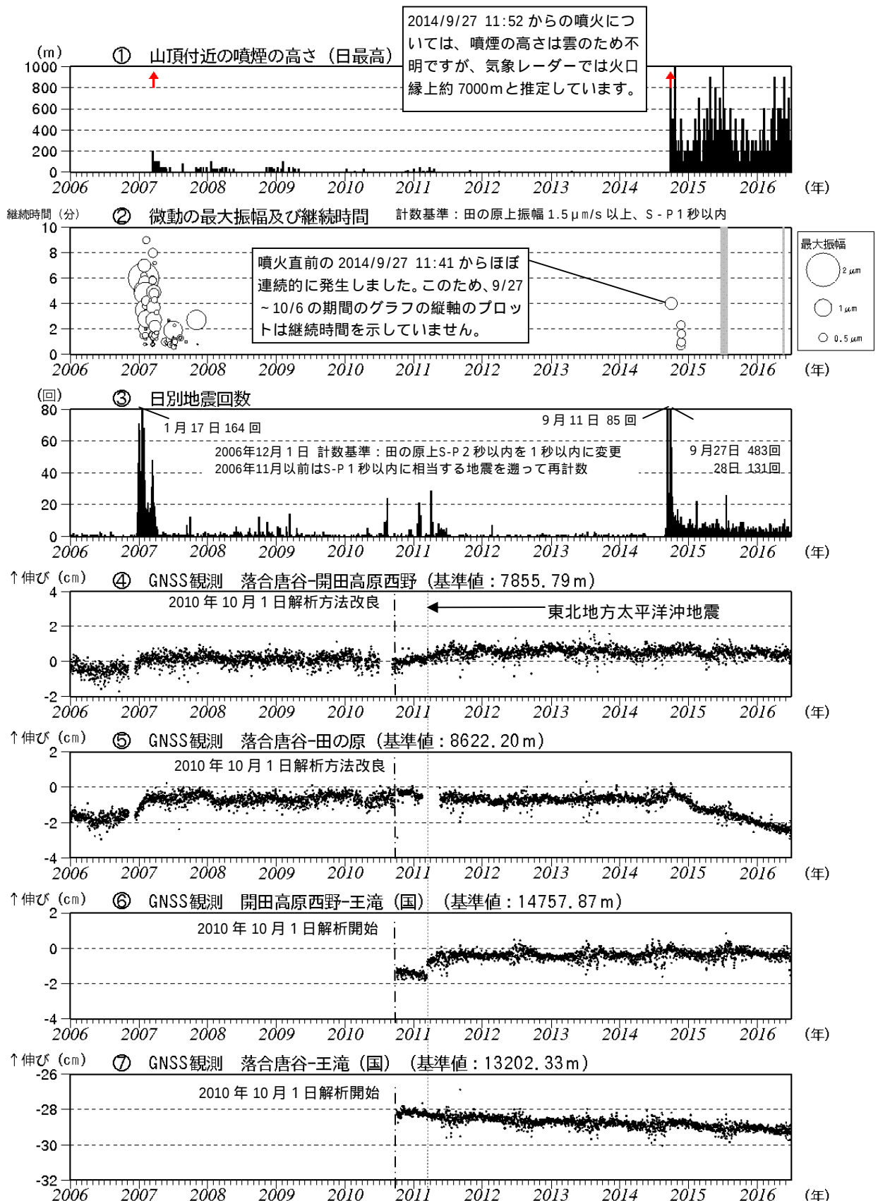
図 4 御嶽山 長期間の火山活動経過図（2006 年 1 月 1 日～2016 年 6 月 30 日）
