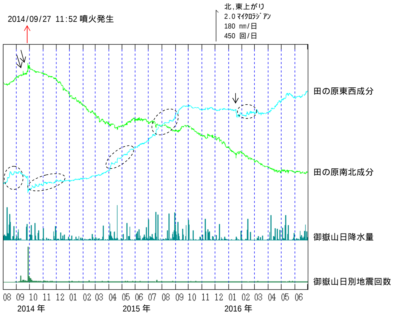
図5 御嶽山 田の原観測点（剣ヶ峰山頂の南東約3 km）の傾斜変動 （2014年8月1日～2016年6月30日）
