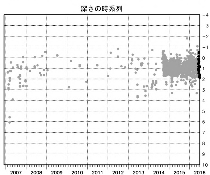
図 2 御嶽山 震源分布図（2006 年 12 月 1 日～2016 年 6 月 30 日）
