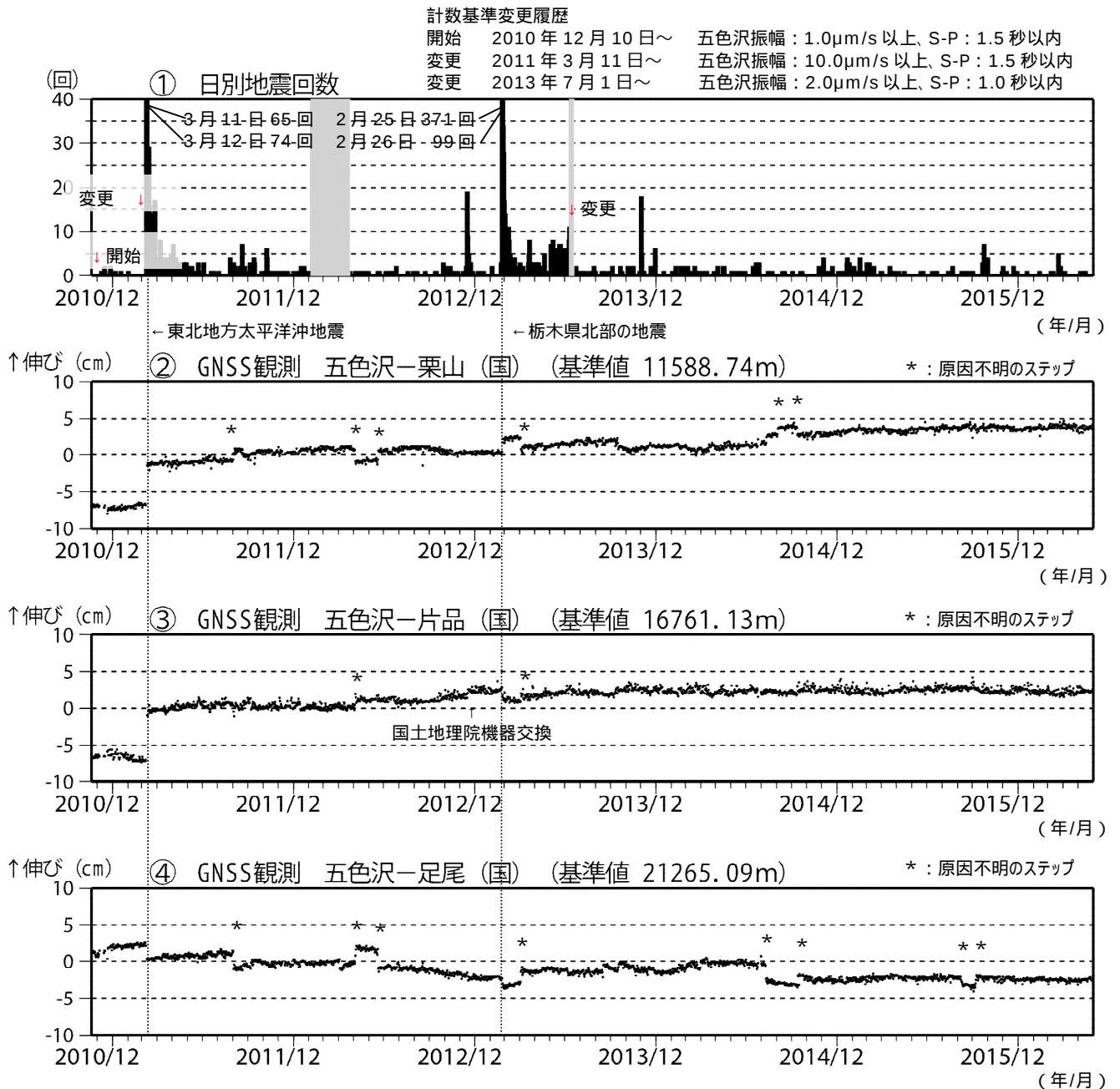
図2 日光白根山 火山活動経過図（2010年11月20日～2016年5月31日）
