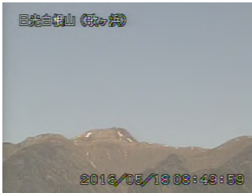
図 1 日光白根山 山頂部の状況（5 月 18 日 歌ヶ浜 うたがはま 遠望カメラによる）
