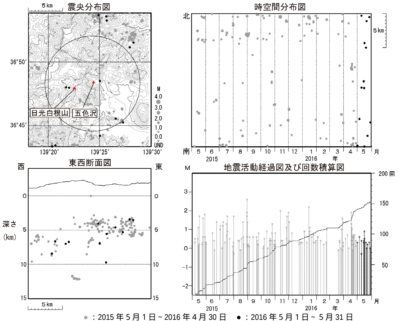
図3 日光白根山 広域地震観測網による山体・周辺の地震活動(2015年5月1日～2016年5月31日) ・震央分布図中の円は図2 - の計数対象地震（五色沢でS - P時間1秒以内）のおよその範囲を示しています。 ・M（マグニチュード）は地震の規模を表します。 ・図中の震源要素は一部暫定値が含まれており、後日変更することがあります。 ・日光白根山付近を震源とする地震の発生は少なく、地震活動は低調に経過しています。
