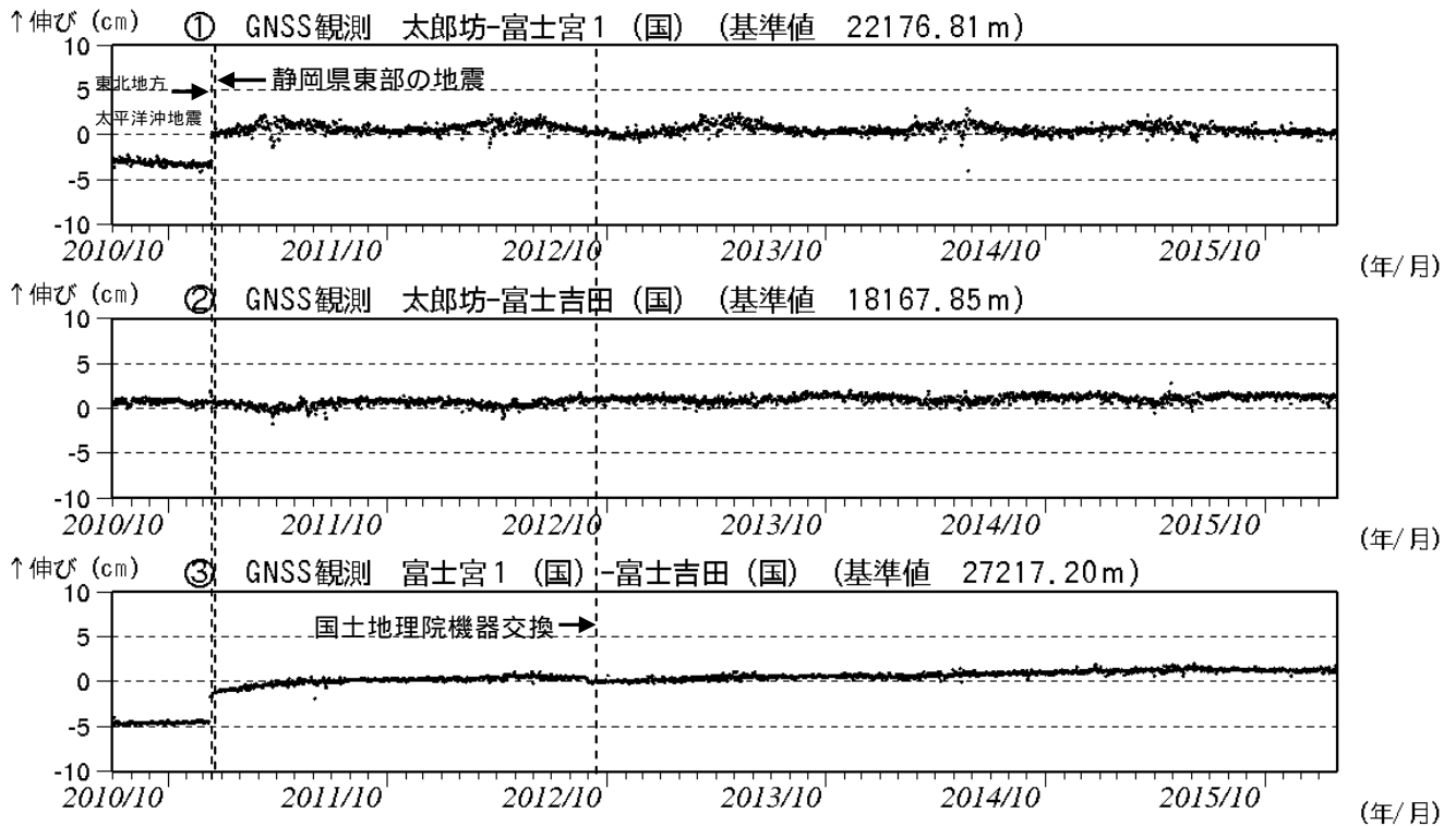
図4 富士山 GNSS 連続観測による基線長変化 (2010 年 10 月 1 日～2016 年 4 月 30 日) (国): 国土地理院
