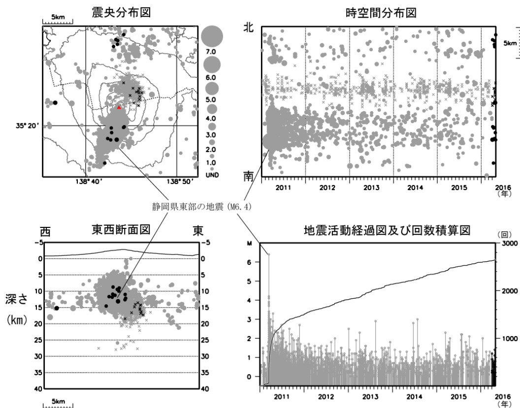
図 3 富士山 広域地震観測網による山体・周辺の地震活動（2011 年 1 月 1 日～2016 年 4 月 30 日）
