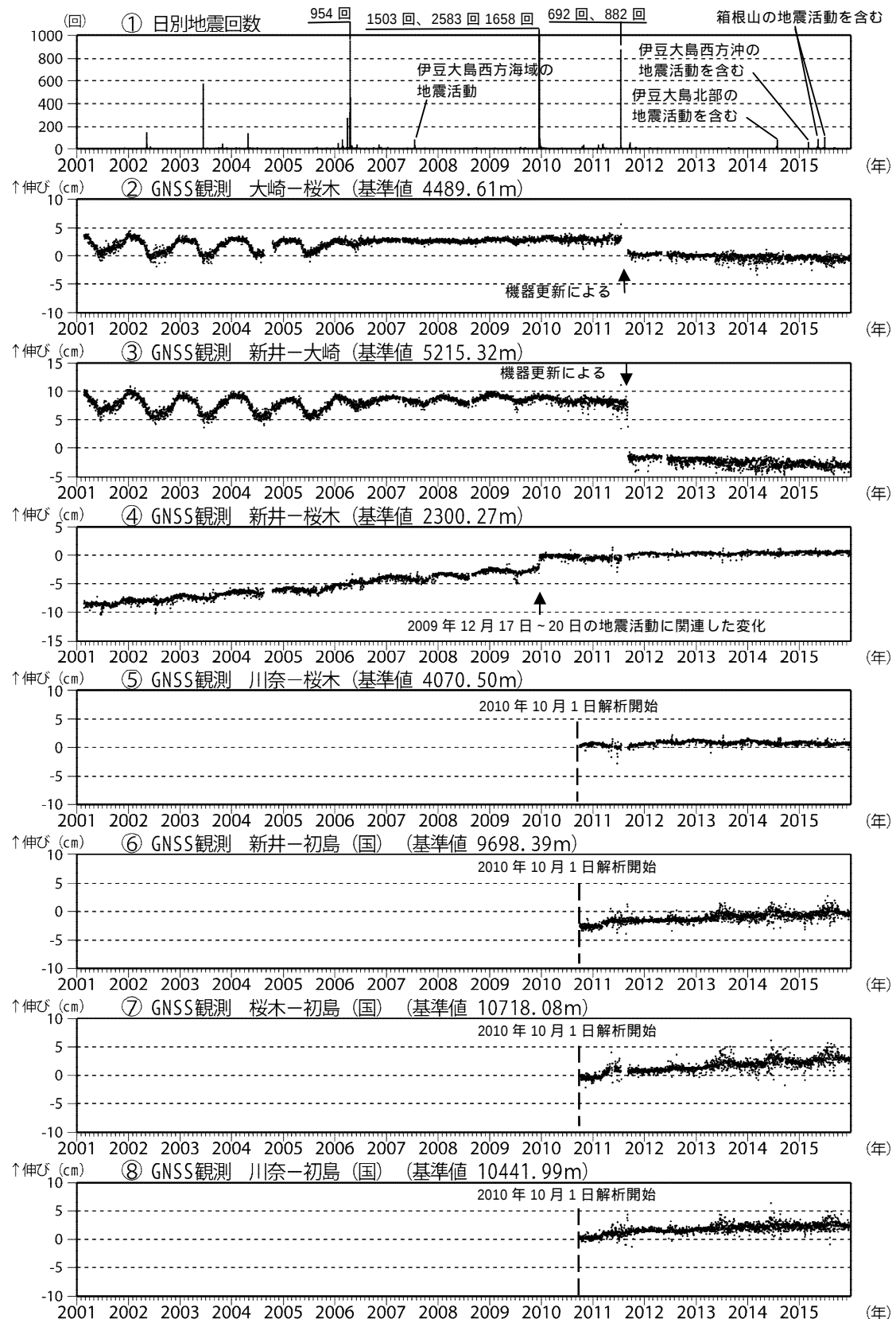
図3 伊豆東部火山群 火山活動経過図（2001年1月1日～2015年12月31日）
