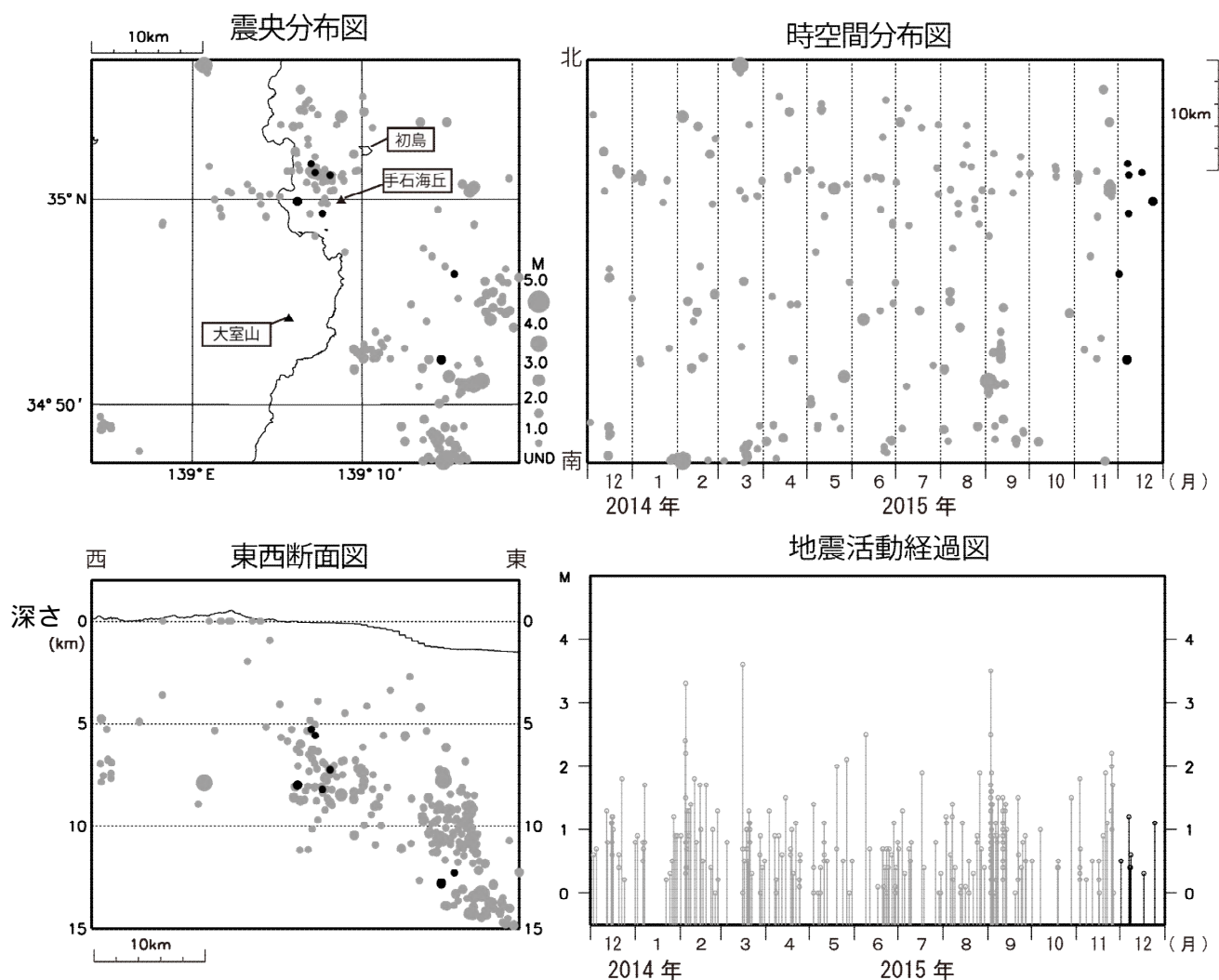
図2 伊豆東部火山群 広域地震観測網による震源分布図（2014年12月1日～2015年12月31日）
