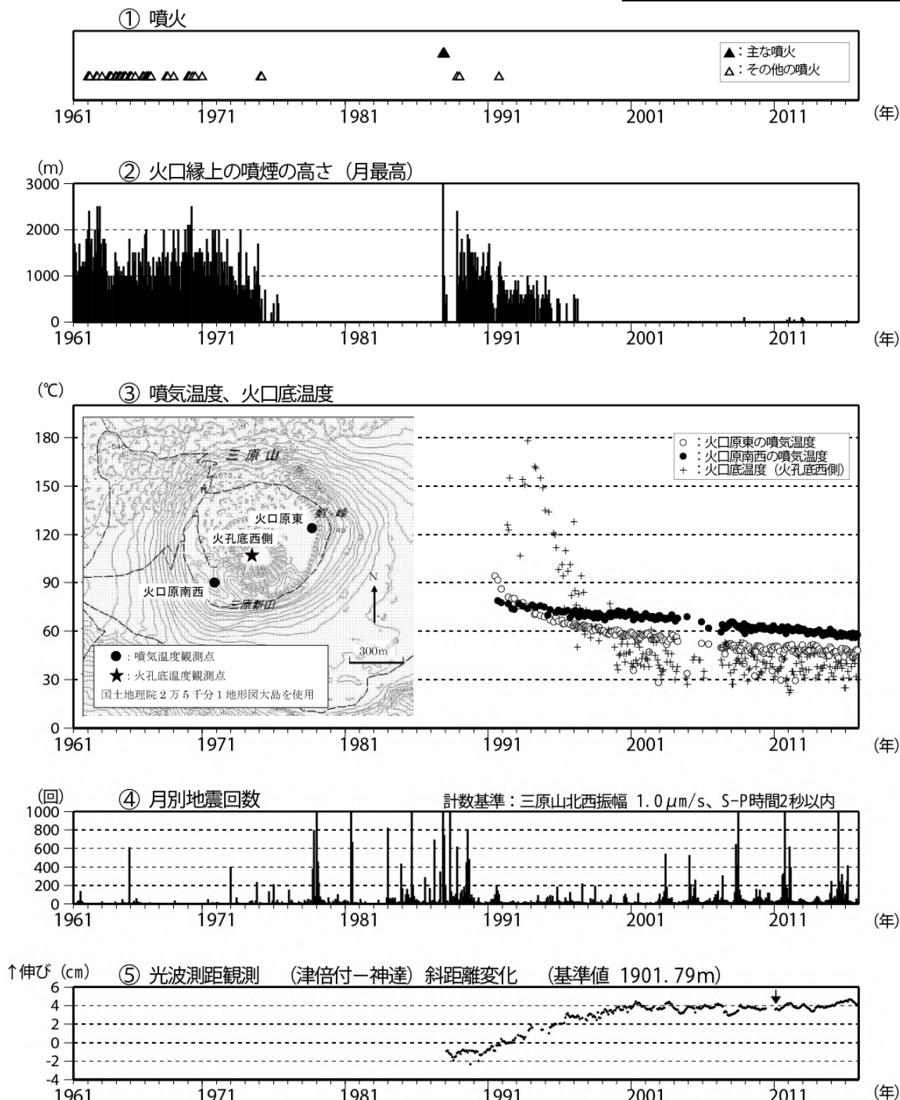
図1 伊豆大島 長期間の火山活動経過図（1961年1月～2015年11月30日）
