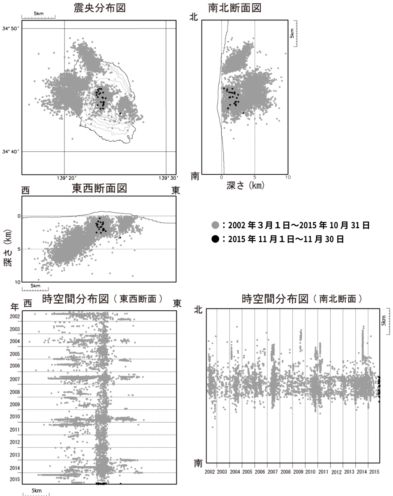
図 4 伊豆大島 震源分布図（2002 年 3 月 1 日～2015 年 11 月 30 日）
