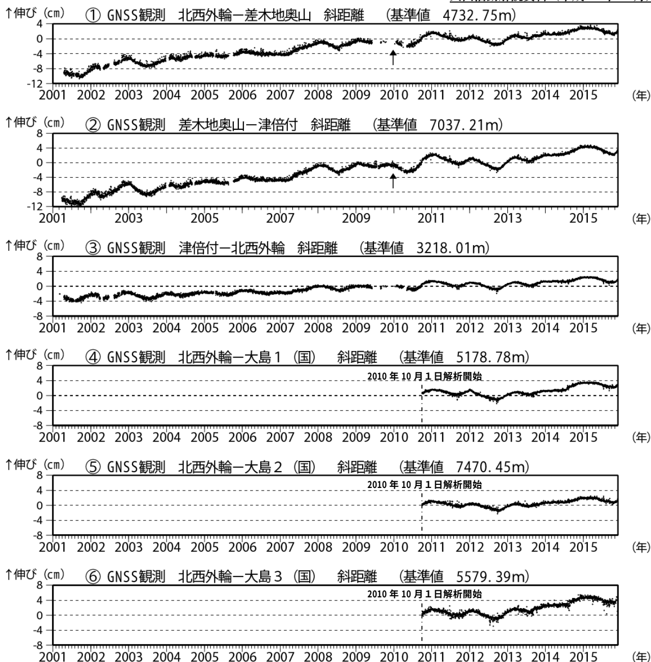
図3 伊豆大島 GNSS連続観測による基線長変化(2001年1月~2015年11月30日)(国):国土地理院
