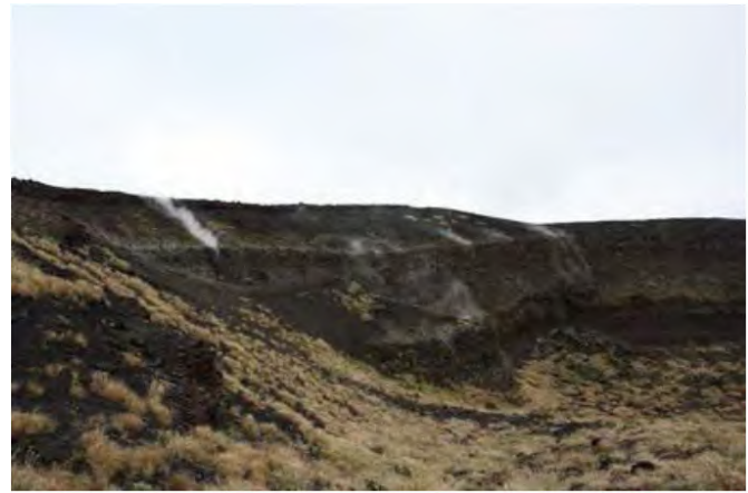
山頂部（11 月 27 日、北西外輪遠望カメラによる） 剣ガ峰付近（11 月 26 日、撮影方向は図 7 参照） 図 5 伊豆大島 三原山山頂部及び山頂火口の状況
