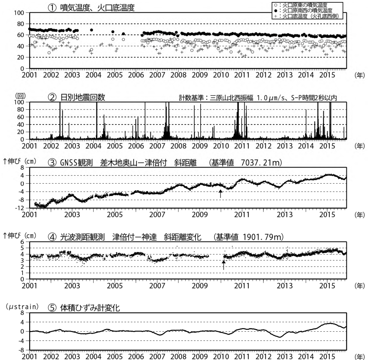
図2 伊豆大島 最近の火山活動経過図（2001年1月～2015年11月30日）
