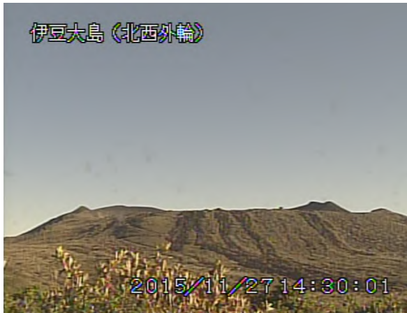
山頂部（11 月 27 日、北西外輪遠望カメラによる） 剣ガ峰付近（11 月 26 日、撮影方向は図 7 参照） 図 5 伊豆大島 三原山山頂部及び山頂火口の状況
