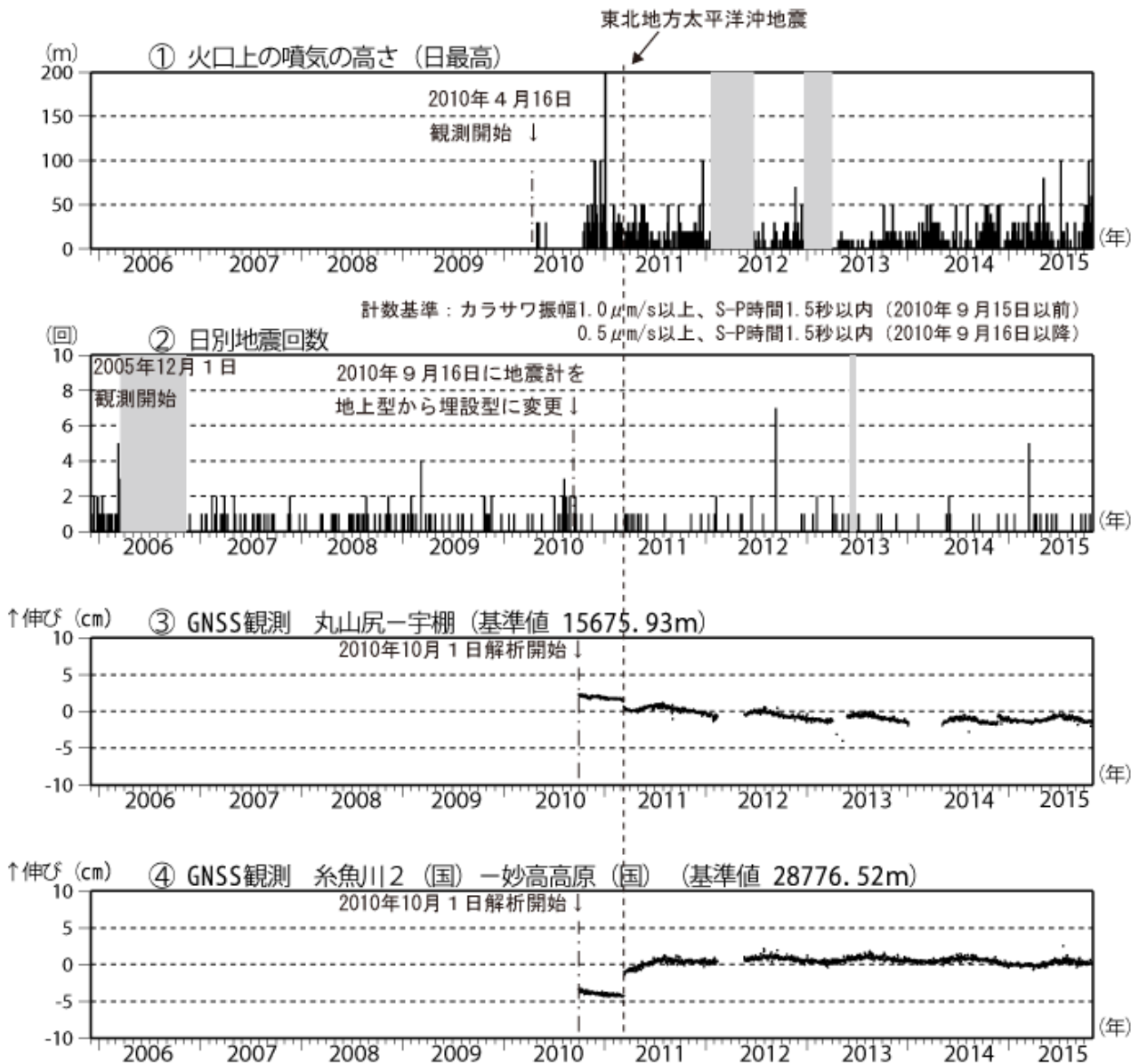
図 3 新潟焼山 火山活動経過図（2005 年 12 月 1 日～2015 年 10 月 31 日）
