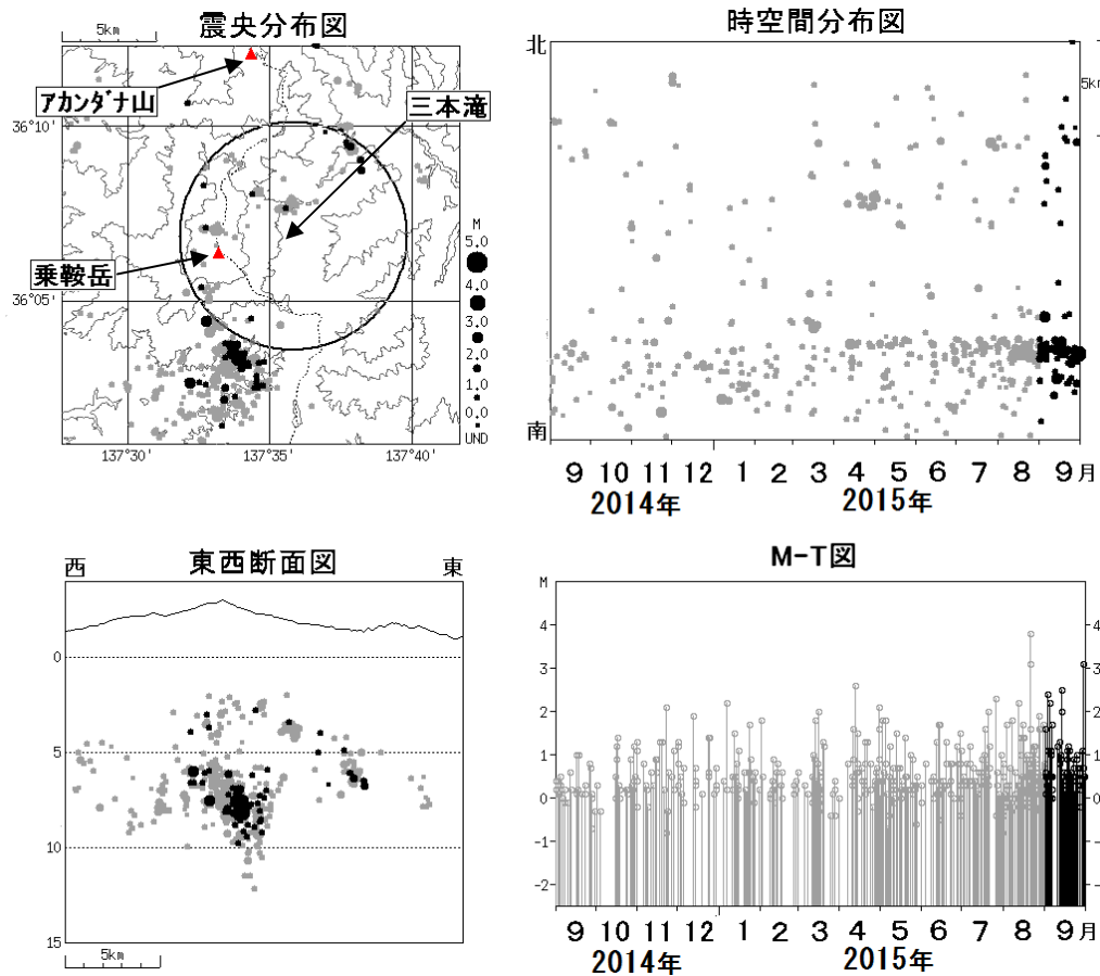
図 3 乗鞍岳 広域地震観測網による山体・周辺の地震活動(2014 年 9 月 1 日～2015 年 9 月 30 日)
