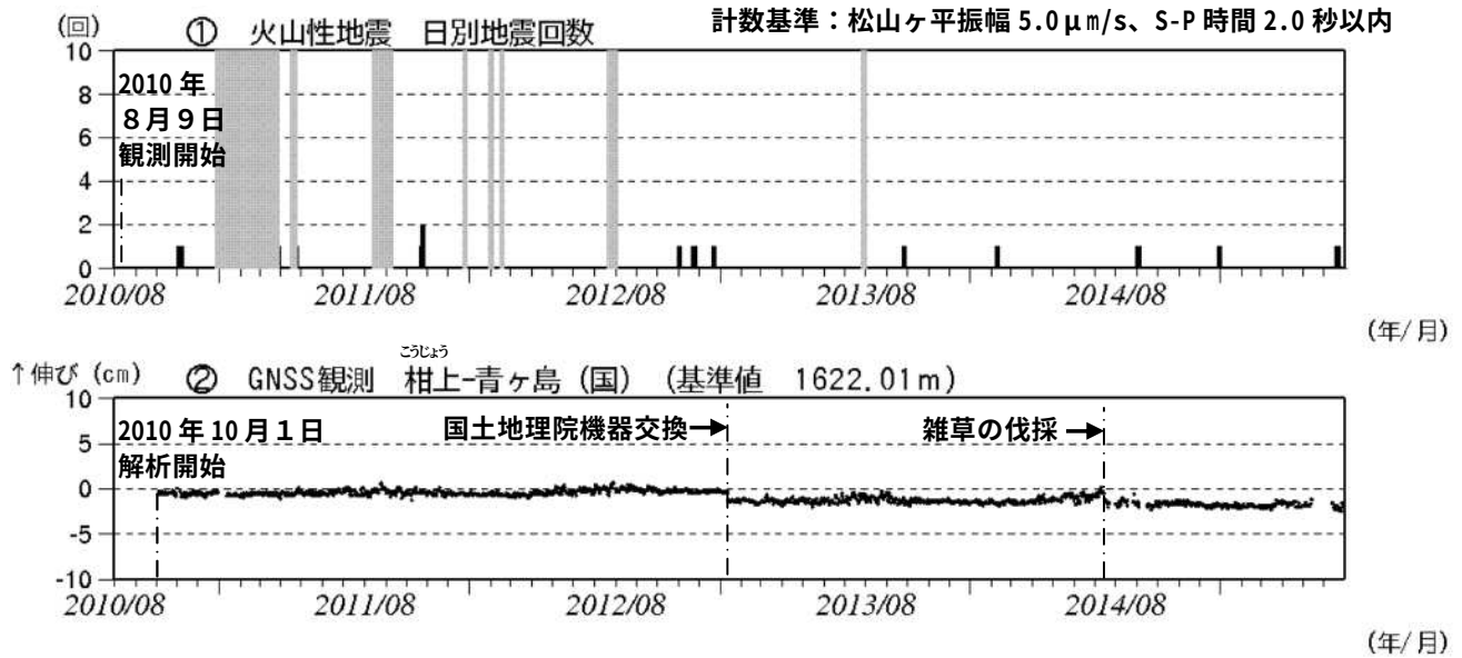
図 2 青ヶ島 火山活動経過図 (2010 年 8 月 9 日～2015 年 6 月 30 日)
