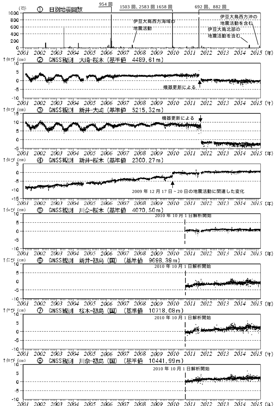
図3 伊豆東部火山群 火山活動経過図（2001年1月1日～2015年3月31日）
