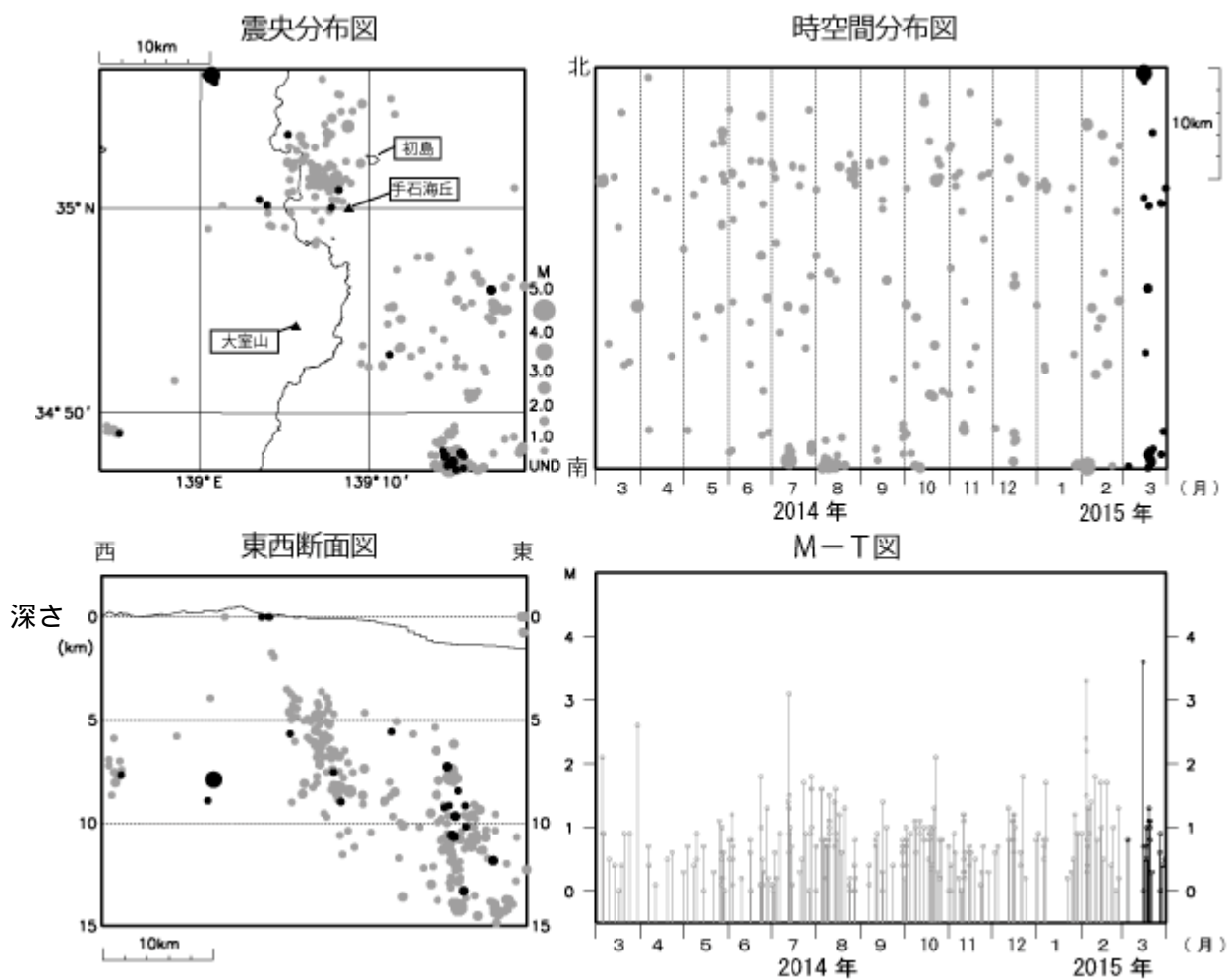
図 2 伊豆東部火山群 広域地震観測網による震源分布図（2014年3月1日～2015年3月31日）
