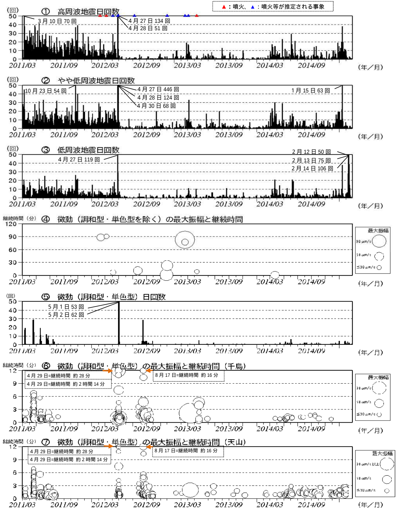
図5 硫黄島 火山活動経過図（2011年3月8日～2015年2月28日）
