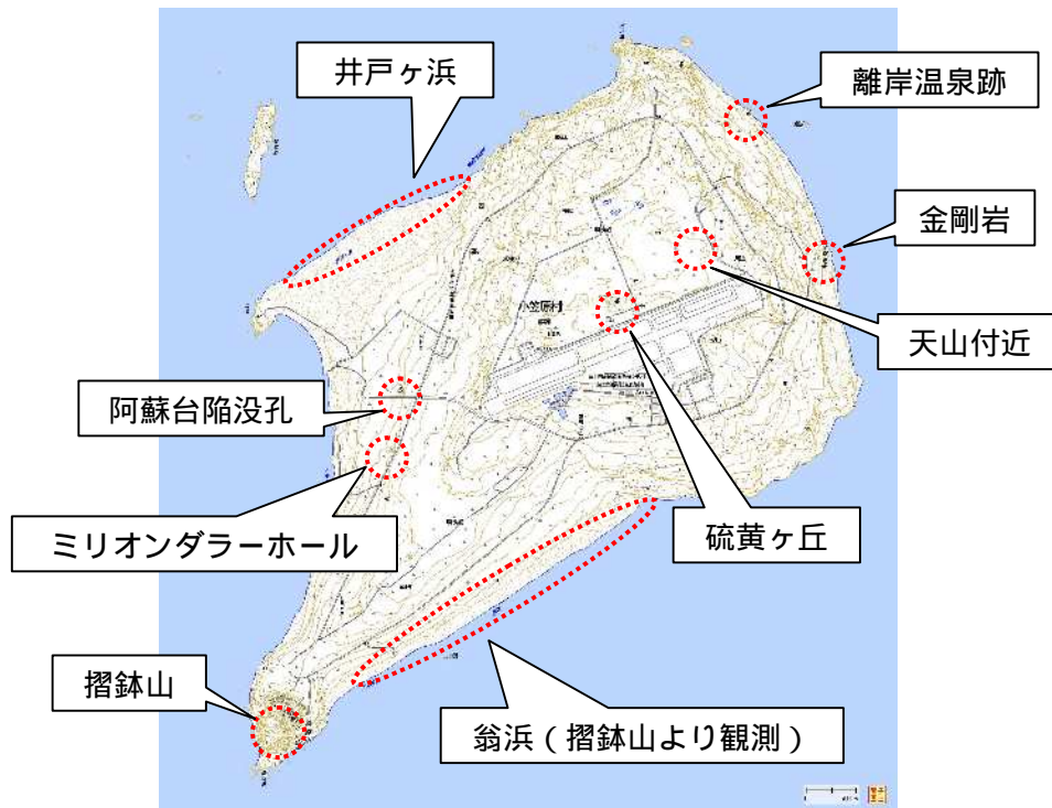
図 9 硫黄島 調査観測を実施した観測地点（2月16日～19日）
