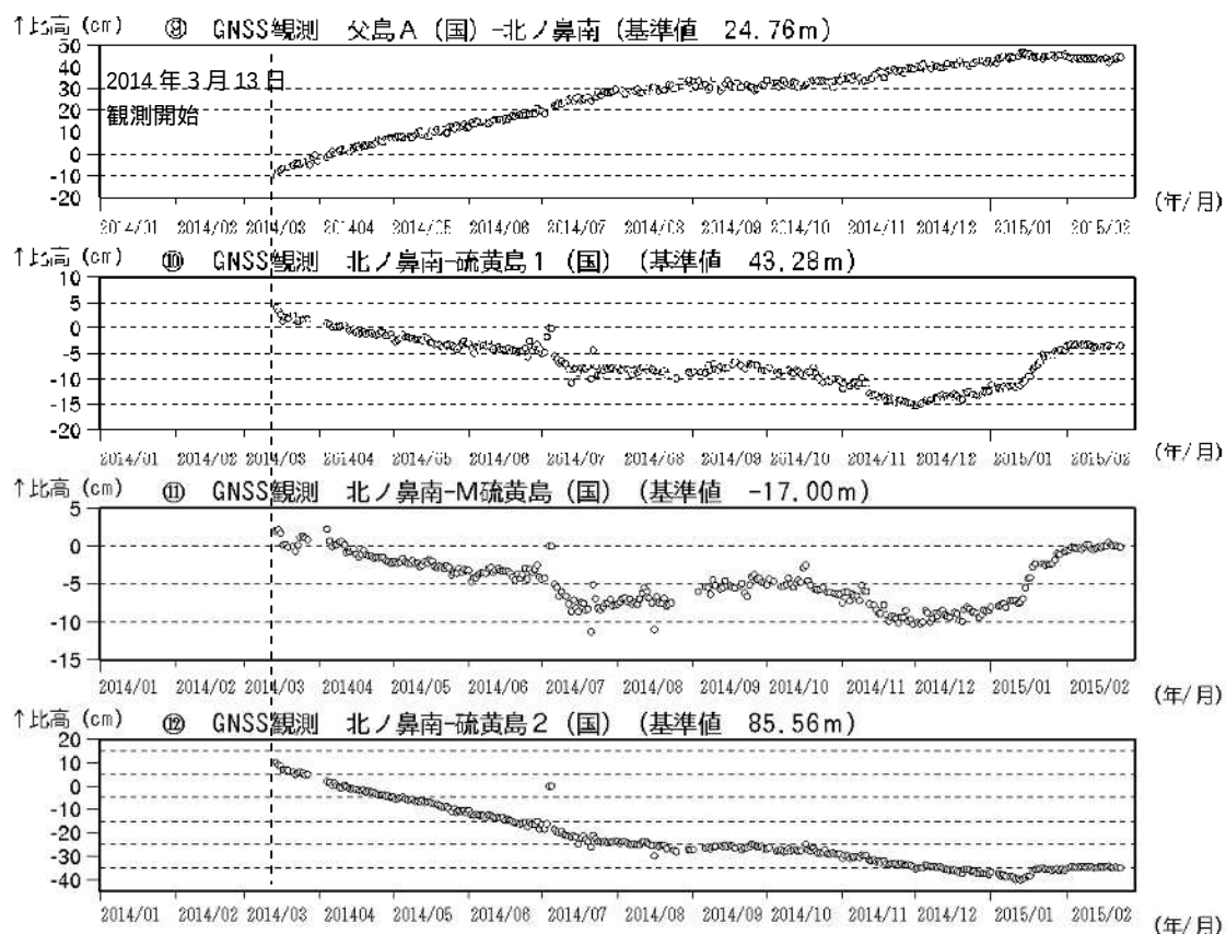
図7 硫黄島 GNSS 2) 観測結果(2014年1月~2015年2月) (国): 国土地理院
