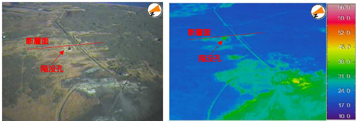
左：可視画像 右：赤外画像 2015 年 2 月 17 日 15 時 36 分撮影
