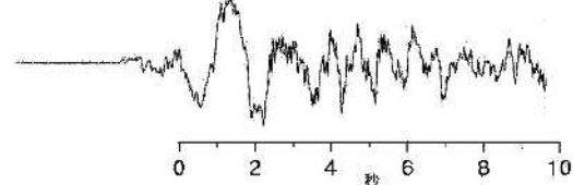
図 5 浅間山で見られる火山性地震の特徴と波形例
