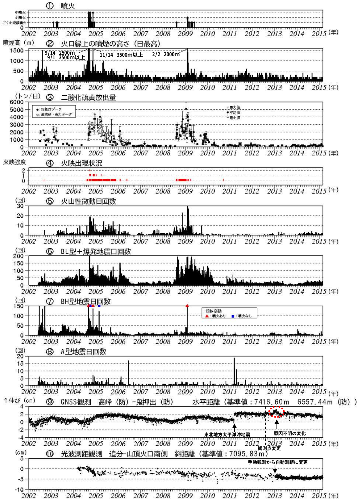
図3 浅間山 火山活動経過図 (2002年1月1日～2015年2月28日)
