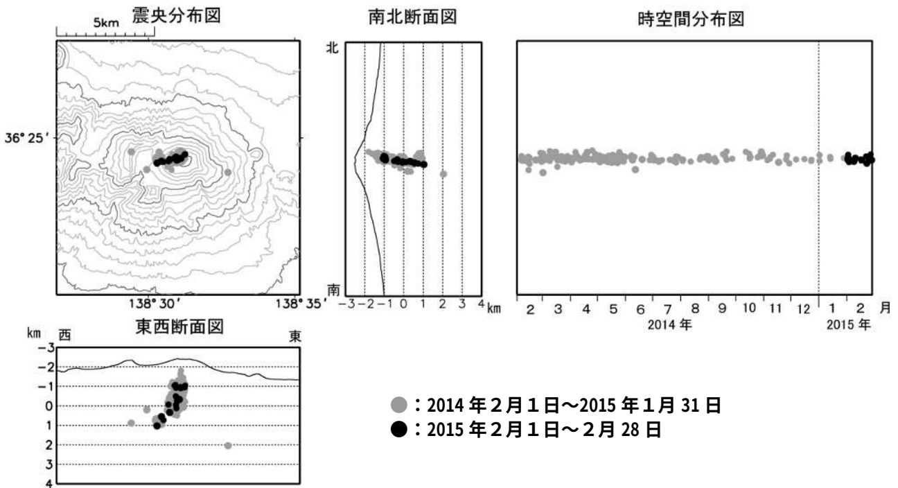
図 4 浅間山 震源分布図（2014 年 2 月 1 日～2015 年 2 月 28 日）
