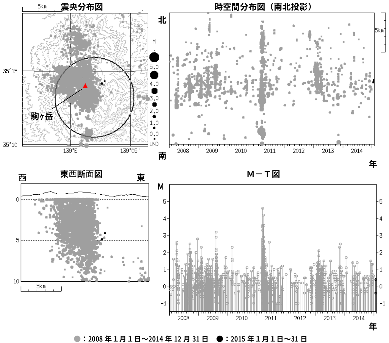
図5 箱根山 広域地震観測網による山体周辺の震源分布図（2008 年 1 月 1 日～2015 年 1 月 31 日） M（マグニチュード）は地震の規模を表します。 図中の震源要素は一部暫定値が含まれており、後日変更することがあります。 震源分布図の円は、駒ヶ岳観測点（温）を中心とした半径 5 km の範囲を示しています。
