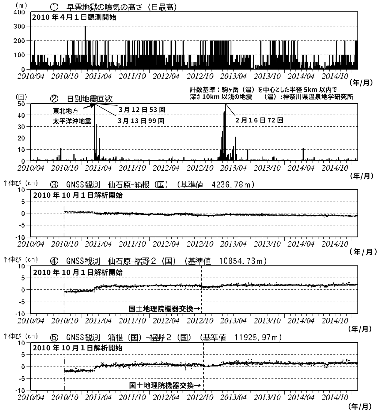
図4 箱根山 火山活動経過図（2010年4月1日～2015年1月31日）
