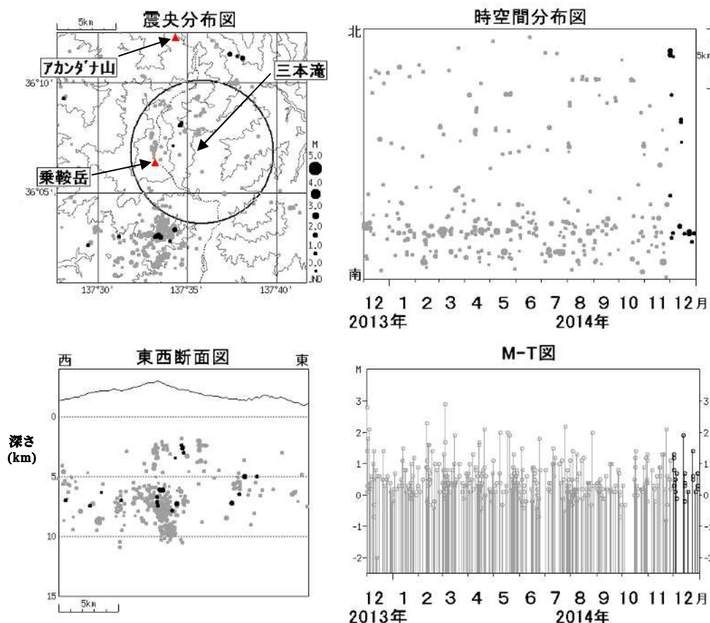
図3 乗鞍岳 広域地震観測網による山体・周辺の地震活動(2013年12月1日～2014年12月31日)
