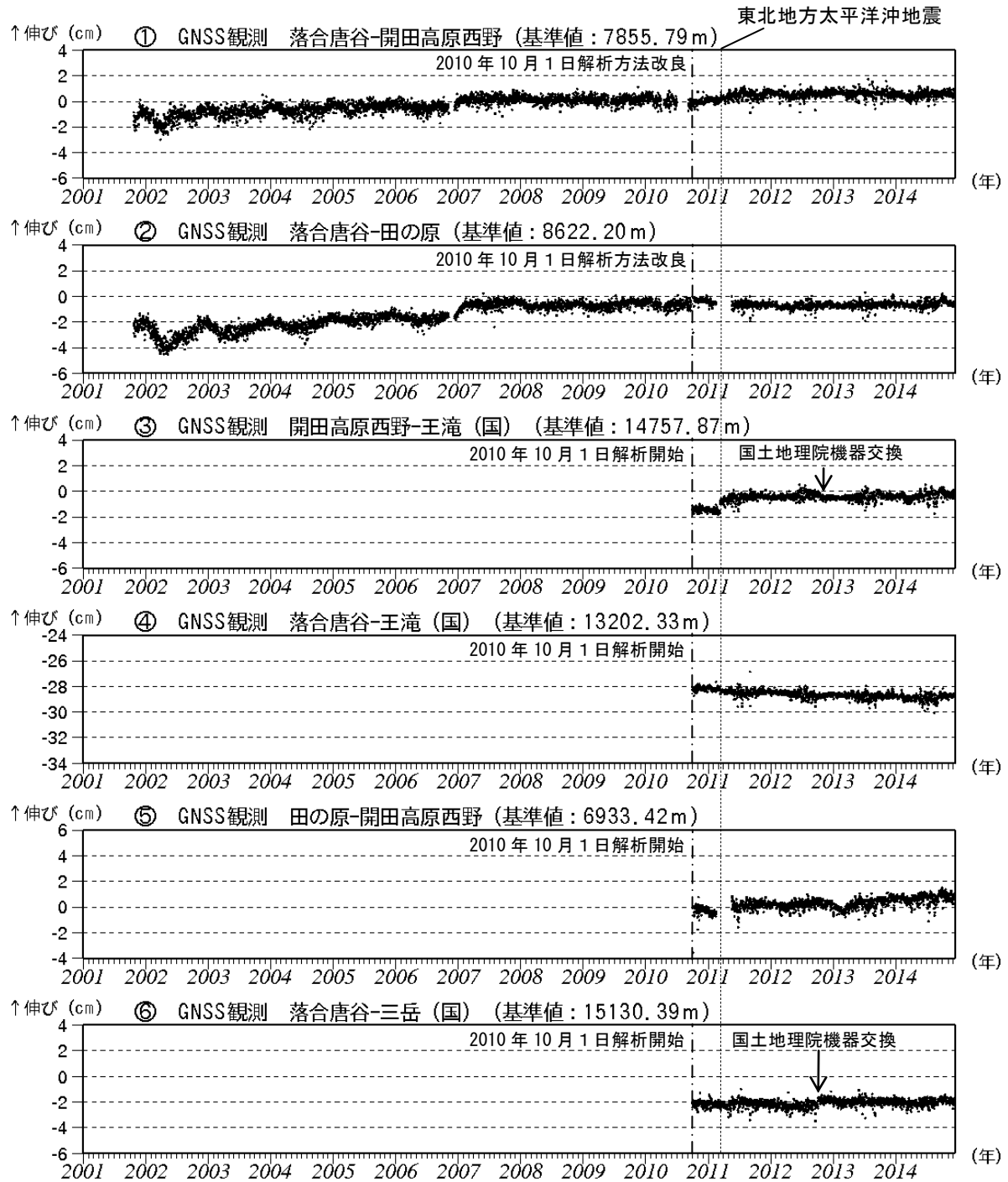
図3 御嶽山 GNSS連続観測による基線長の長期変化 (2001年1月1日～2014年12月12日)
