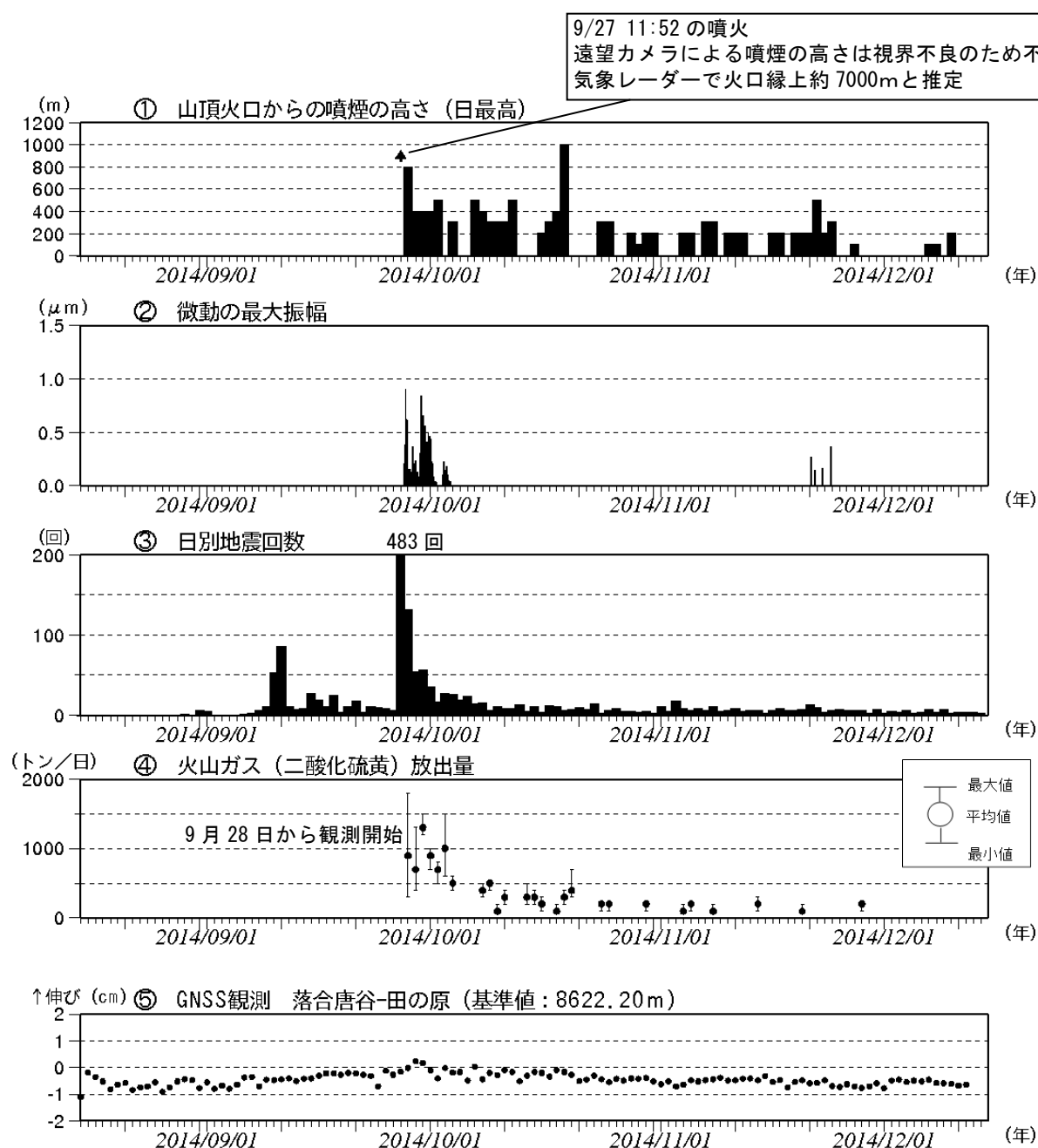
図2 御嶽山 日別活動状況（2014年8月15日～12月14日（速報値含む））
