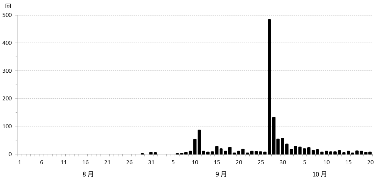
図 2 御嶽山 日別地震回数（2014 年 8 月 1 日～10 月 20 日（速報値含む）） ・火山性地震は噴火直後に比べて減少し、やや少ない状態で推移しています。
