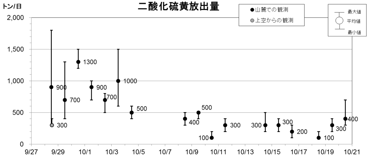
図 1 御嶽山 火山ガス（二酸化硫黄）観測結果（9 月 28 日～10 月 20 日） ・昨日（20 日）に山麓で実施した火山ガス観測では、二酸化硫黄の放出量は、1 日あたり およそ 300～700 トン（速報値）で、噴火発生直後に比べやや少ない状態が続いています。
