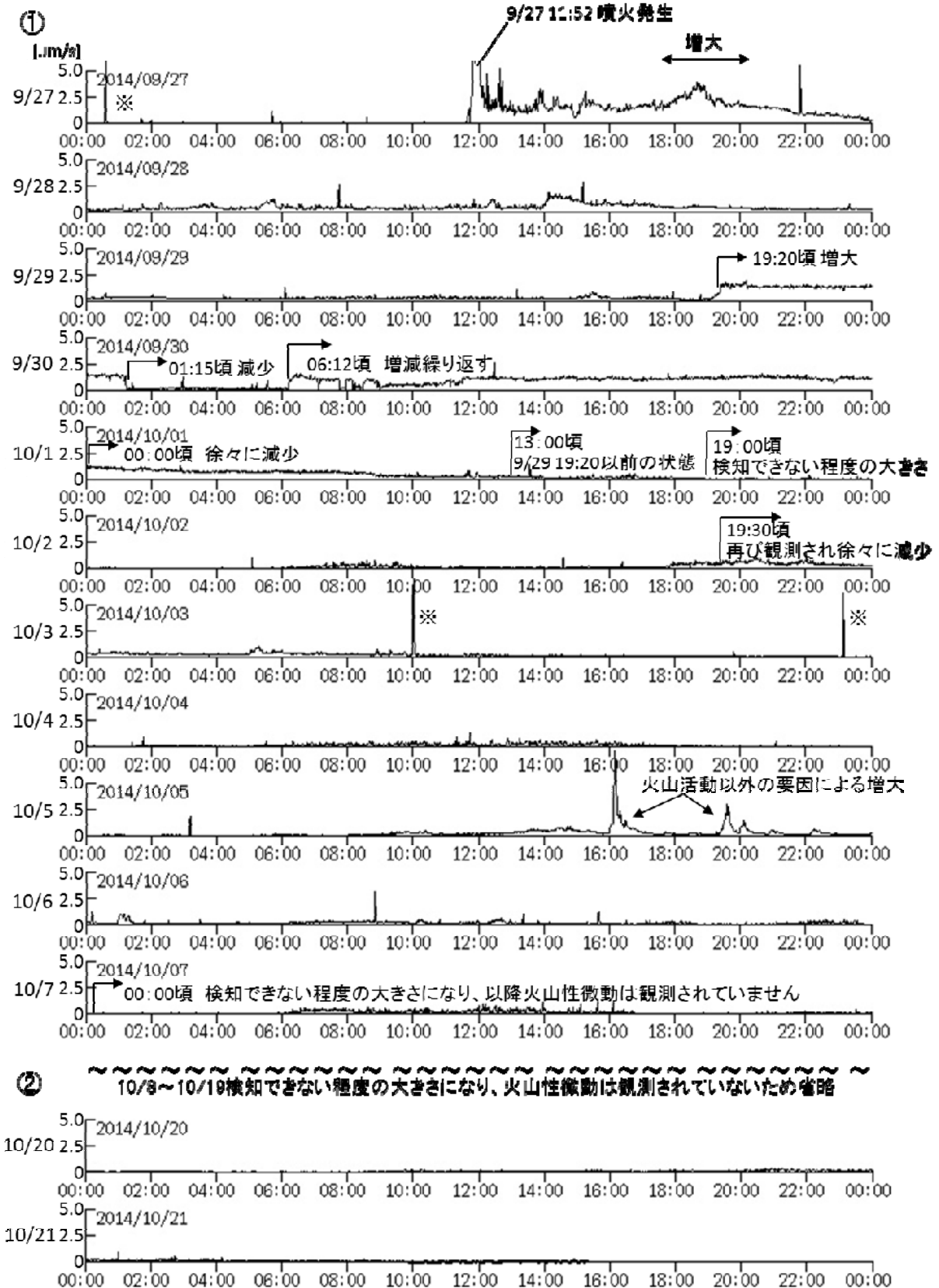
図3 御嶽山 田の原上観測点（剣ヶ峰の南東約2km）の上下動地震波形の1分間振幅平均値の推移 期間 2014年9月27日00時～10月7日24時00分 期間 2014年10月20日00時～10月21日15時20分 火山活動以外の地震による ・火山性微動は、検知できない大きさになった10月7日以降は観測されていません。
