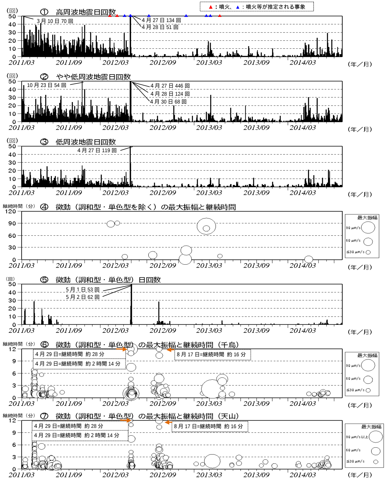
図5 硫黄島 火山活動経過図（2011年3月8日～2014年7月31日）
