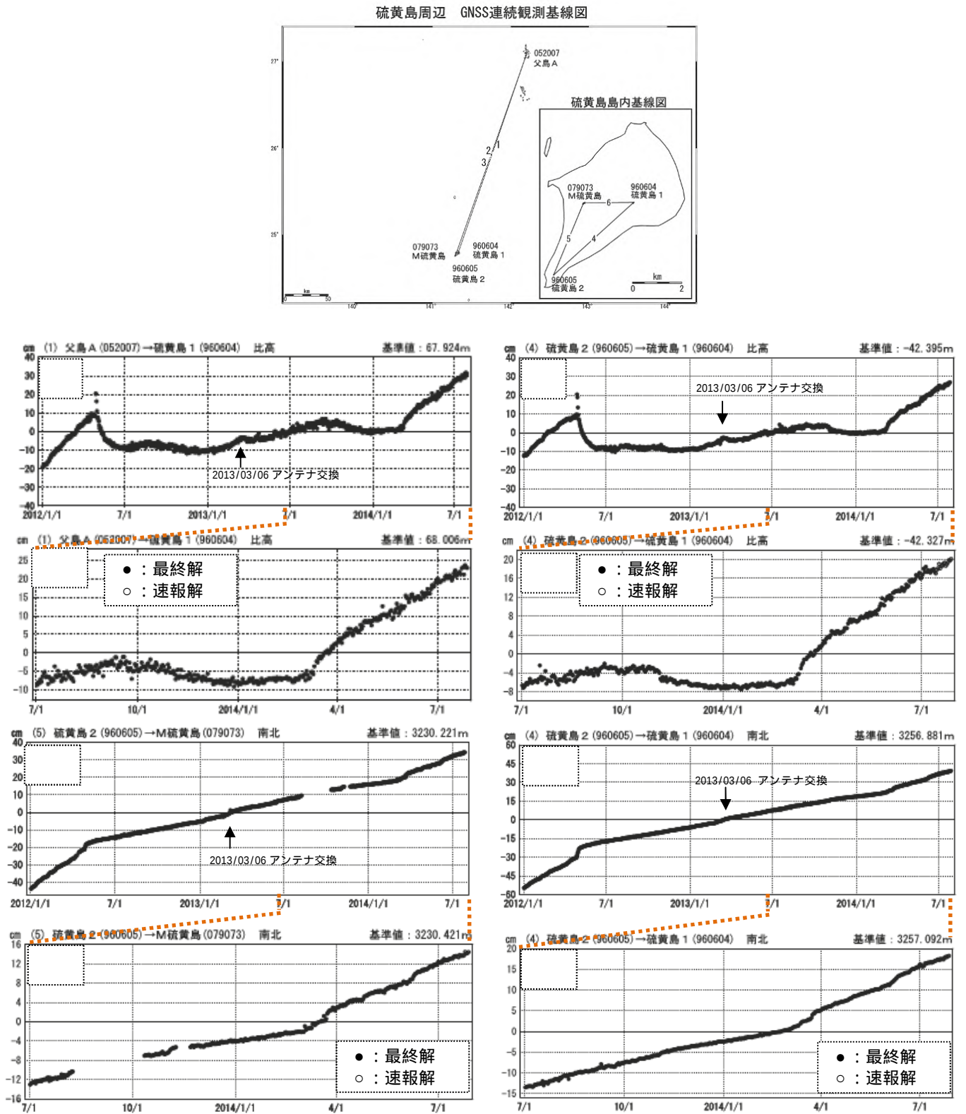
図 6 硫黄島 国土地理院による地殻変動観測結果 1)
