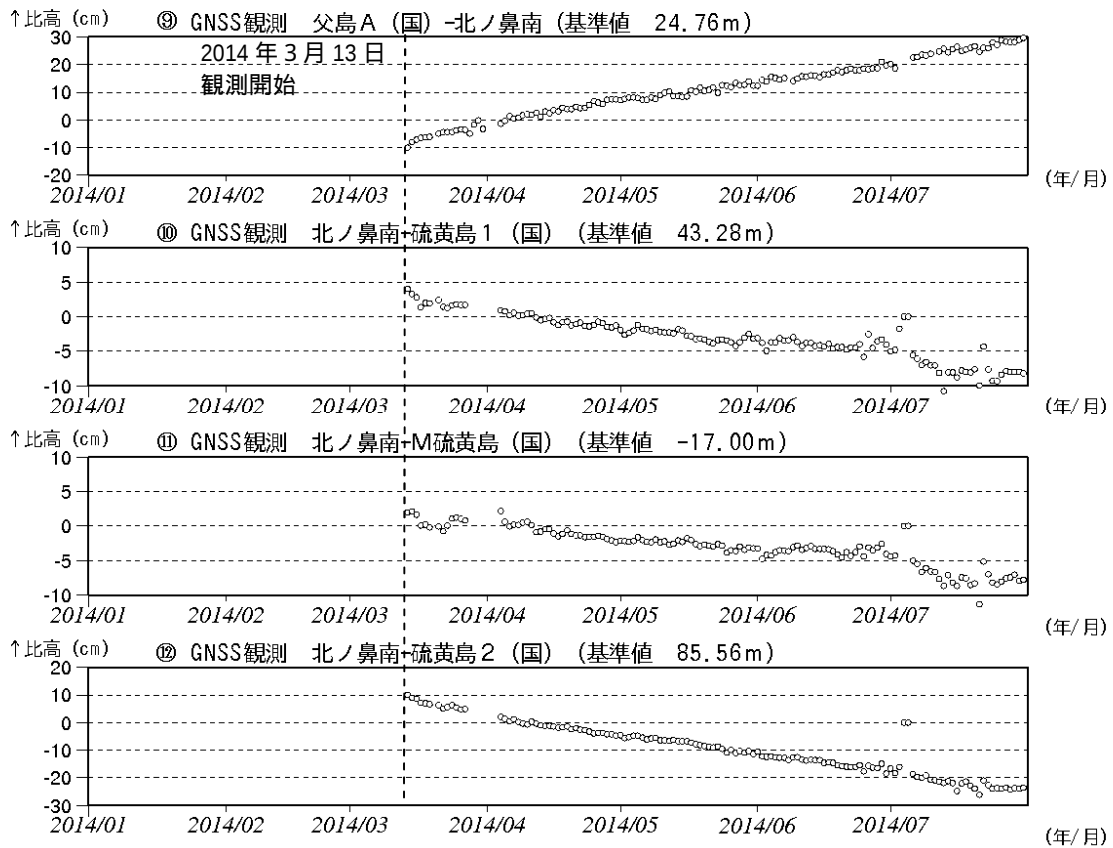
図7 硫黄島 GNSS 2) 観測結果 (2014年1月～7月) (国): 国土地理院
