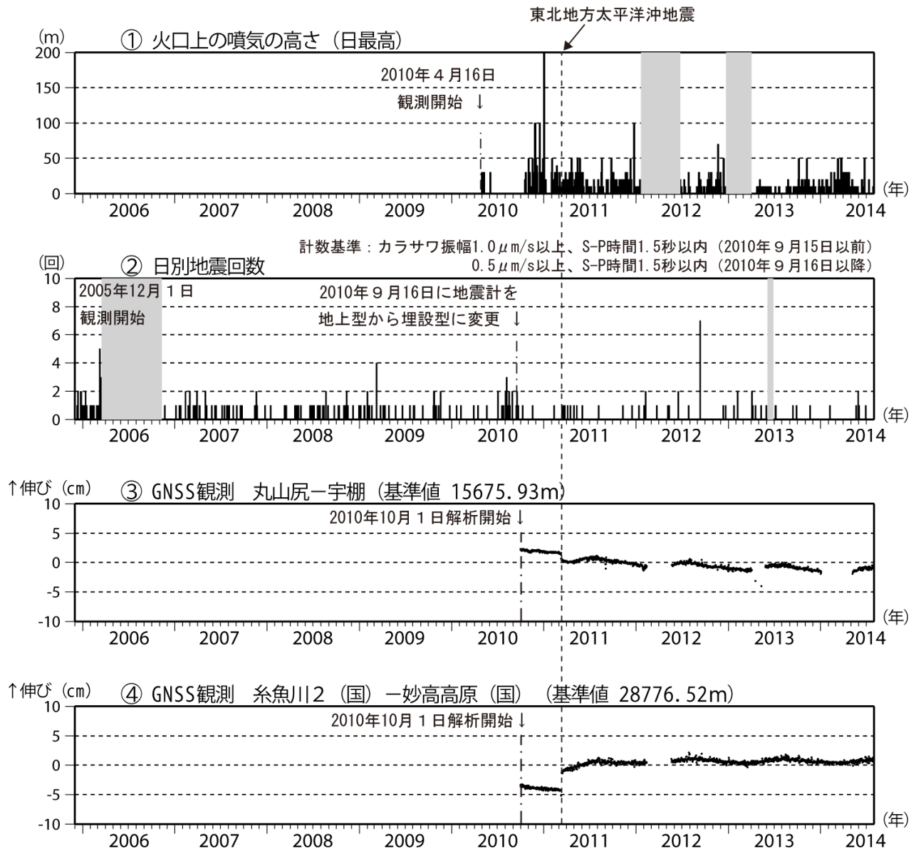
図3 新潟焼山 火山活動経過図（2005年12月1日～2014年7月31日）
