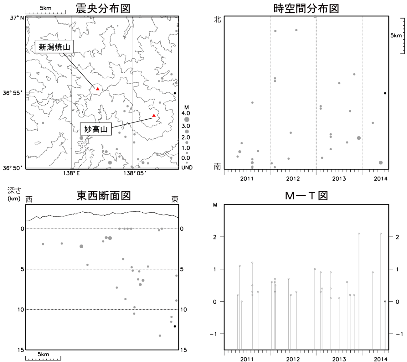
図 4 新潟焼山 広域地震観測網による山体・周辺の地震活動（2011 年 1 月 1 日～2014 年 7 月 31 日）
