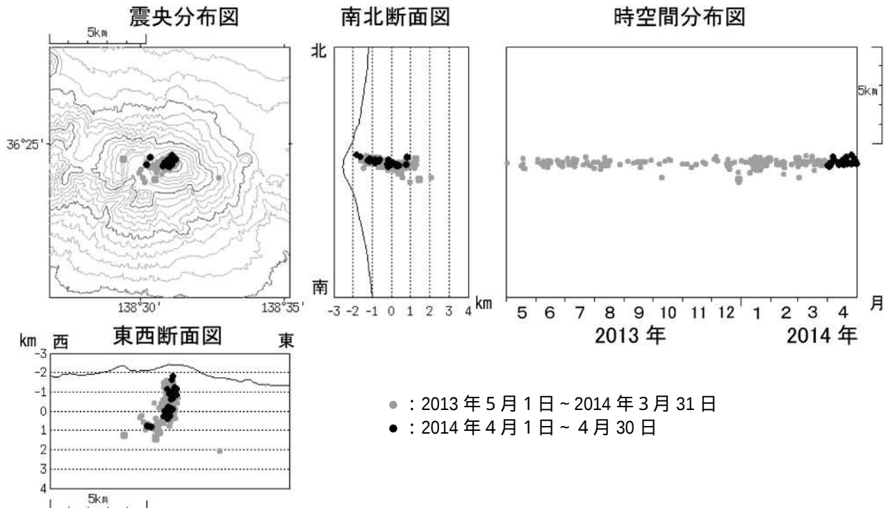
図 6 浅間山 震源分布図（2013 年 5 月 1 日～2014 年 4 月 30 日）
