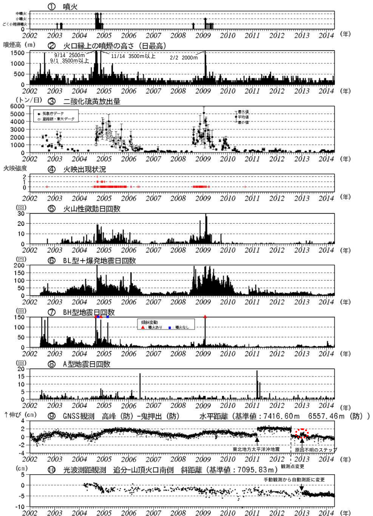
図5 浅間山 最近の火山活動経過図 (2002年1月1日～2014年4月30日)
