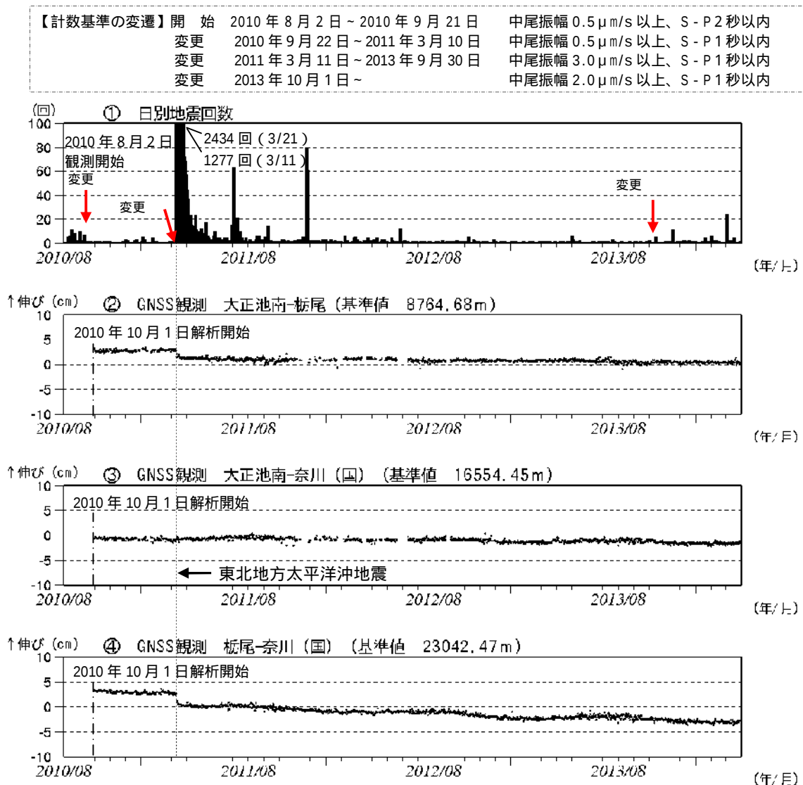
図 3 焼岳 火山活動経過図（2010年 8 月 2 日 ~ 2014年 3 月31日）
