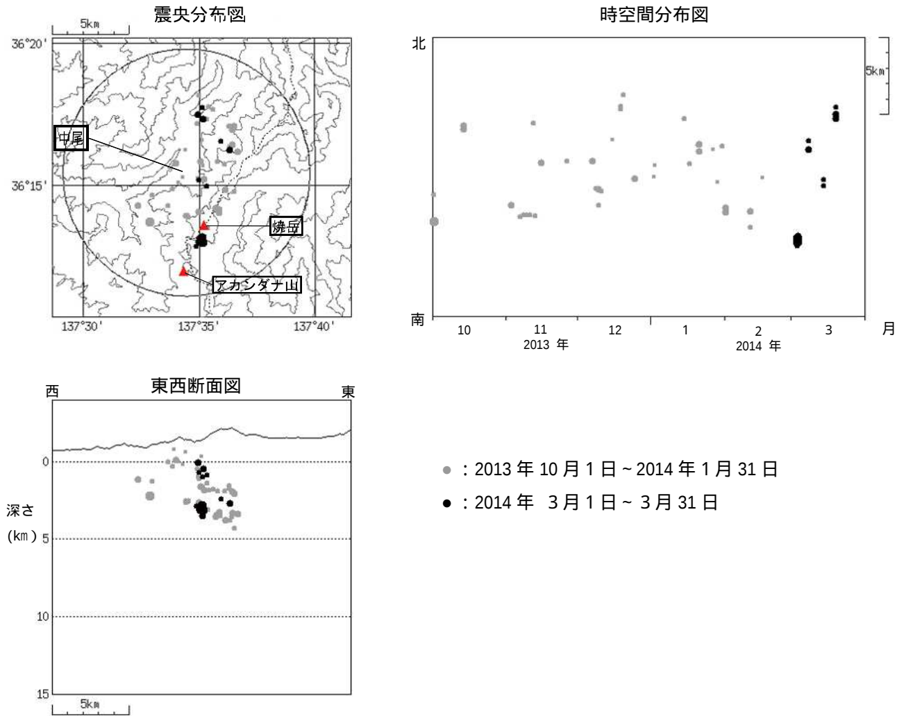
図 4 焼岳 震源分布図（2013 年 10 月 1 日～2014 年 3 月 31 日） 震央分布図中の円は図 3 - の計数対象地震（中尾で S - P 時間 1 秒以内）のおよその範囲を示します。
