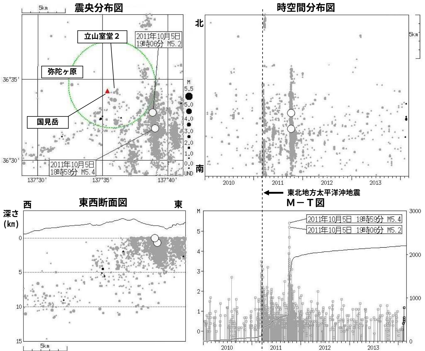
図2 弥陀ヶ原 広域地震観測網による山体・周辺の地震活動（2010年1月1日～2014年2月28日）
