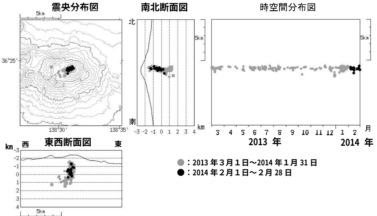
図 4 浅間山 震源分布図（2013 年 3 月 1 日～2014 年 2 月 28 日）
