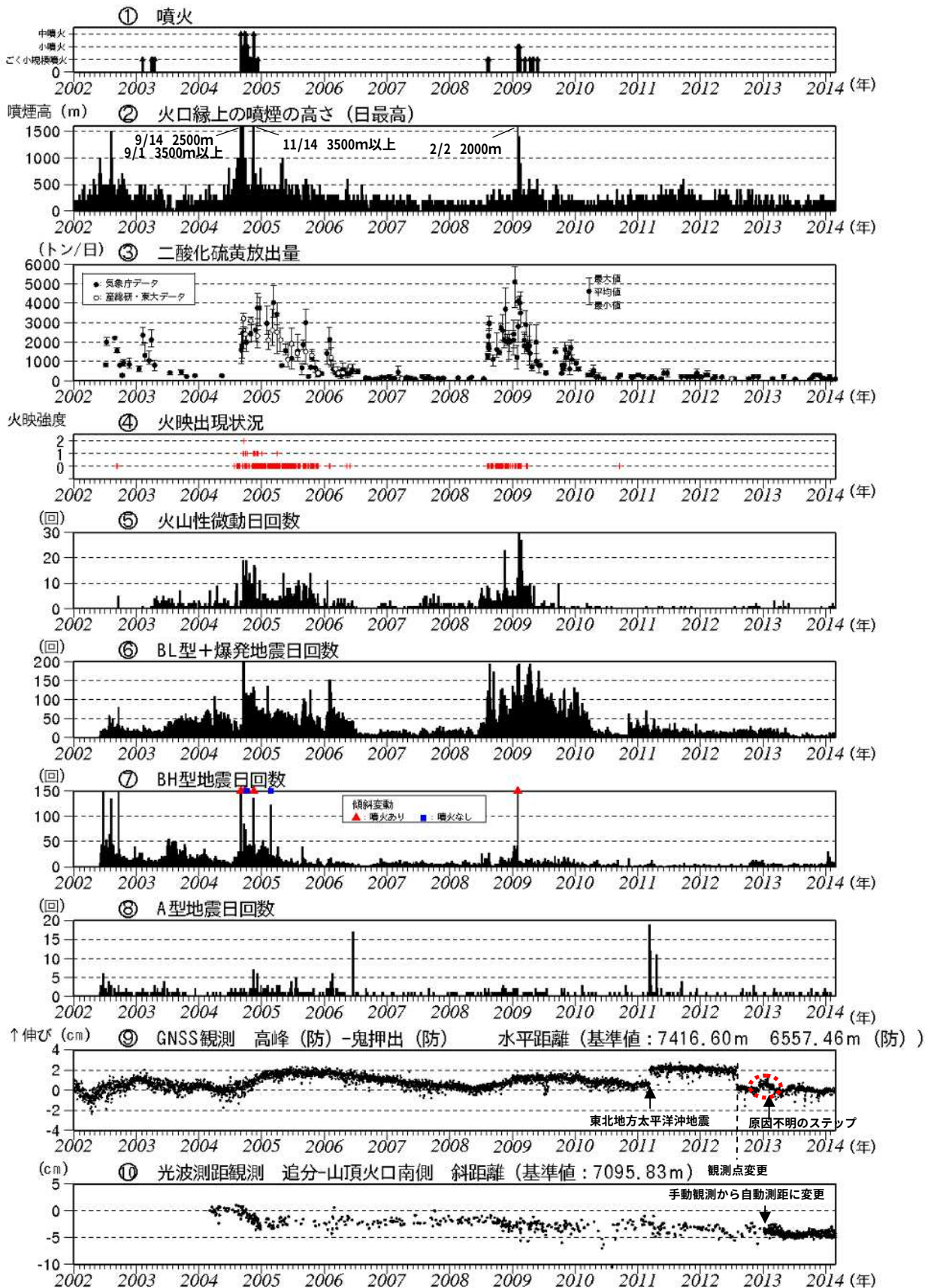
図3 浅間山 最近の火山活動経過図 (2002年1月1日～2014年2月28日)
