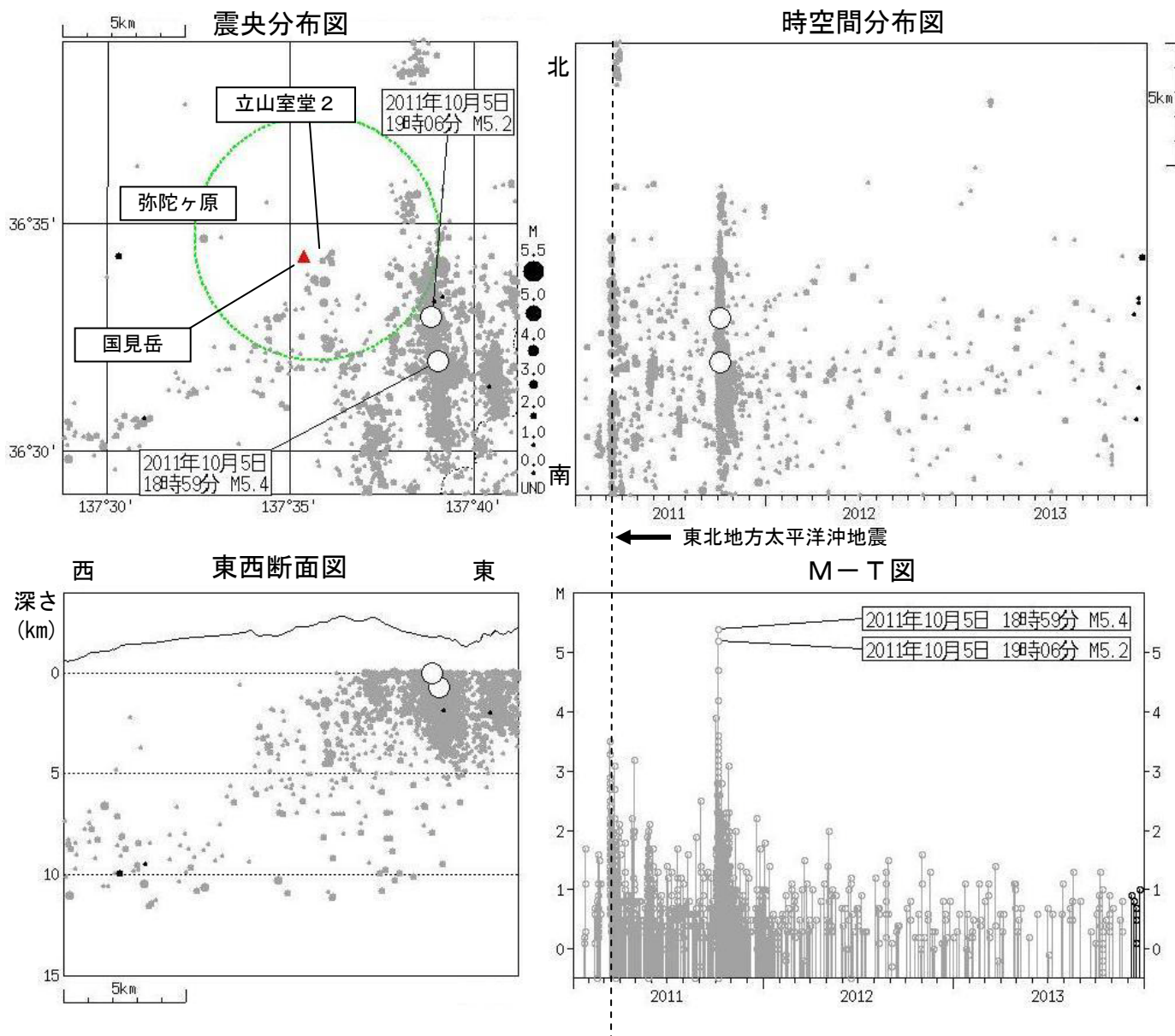
図2 弥陀ヶ原 広域地震観測網による山体・周辺の地震活動（2011年1月1日～2013年12月31日）
