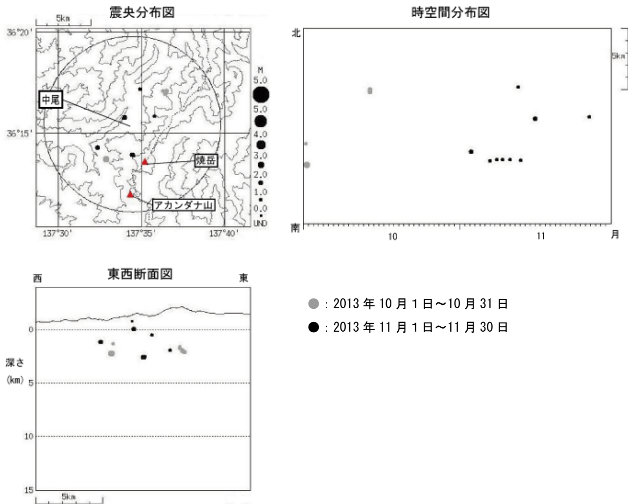
図 4 焼岳 震源分布図（2013 年 10 月 1 日～11 月 30 日）
