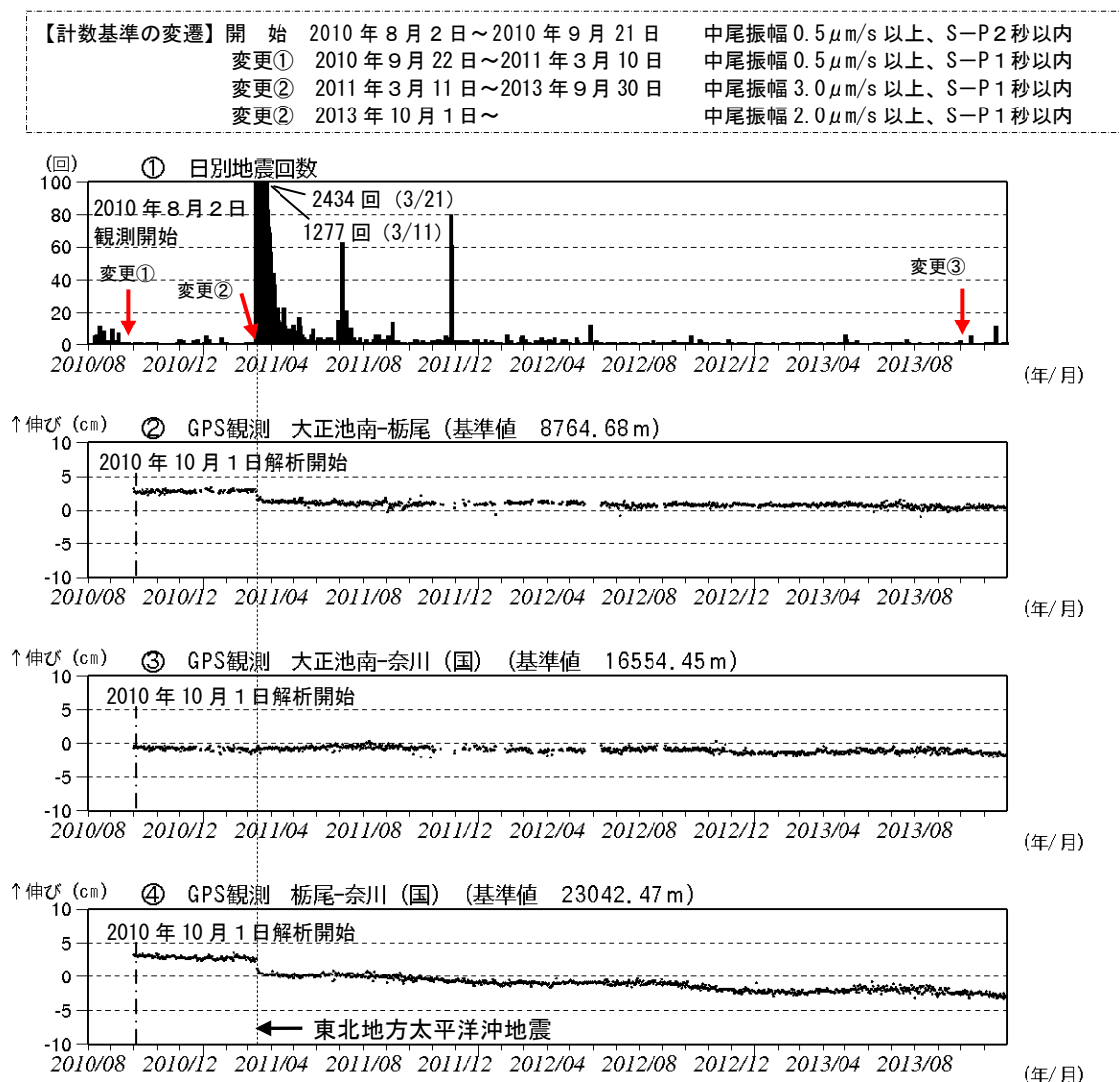
図 3 焼岳 火山活動経過図 (2010年 8 月 2 日～2013年11月30日)
