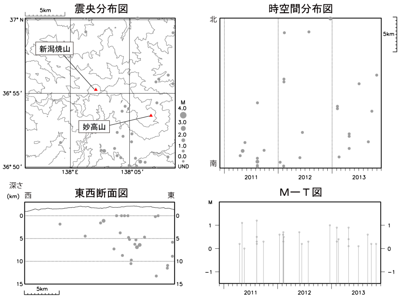
図 4 新潟焼山 広域地震観測網による山体・周辺の地震活動（2010 年 12 月 1 日～2013 年 11 月 30 日）
