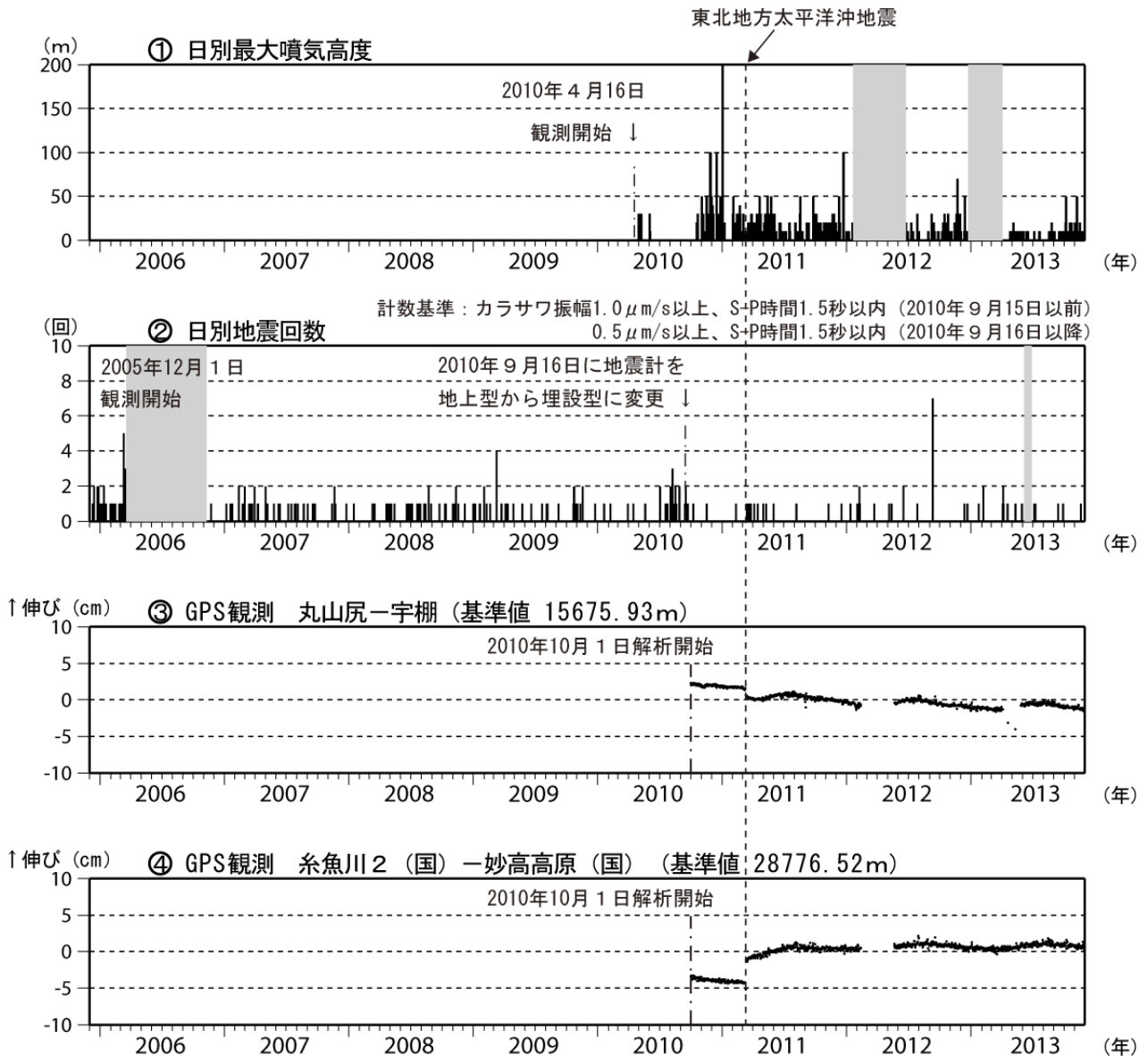
図3 新潟焼山 火山活動経過図（2005年12月1日～2013年11月30日）
