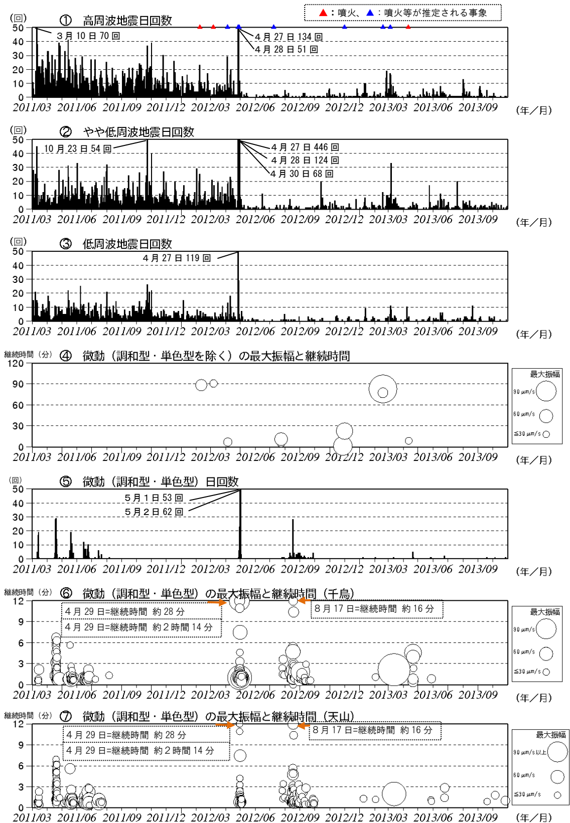
図5 硫黄島 火山活動経過図（2011年3月8日～2013年10月31日）
