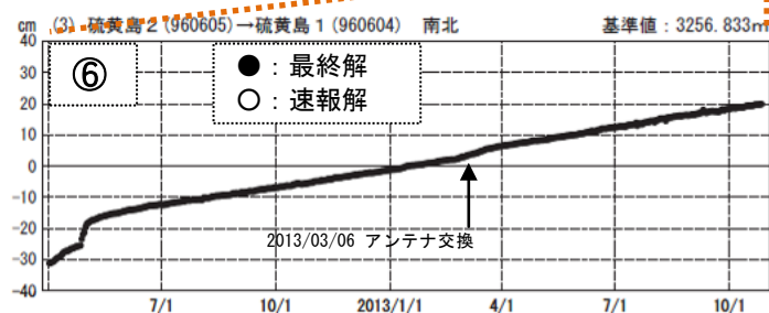
図6 硫黄島 国土地理院による地殻変動観測結果 1) (2010年10月1日～2013年10月27日)
