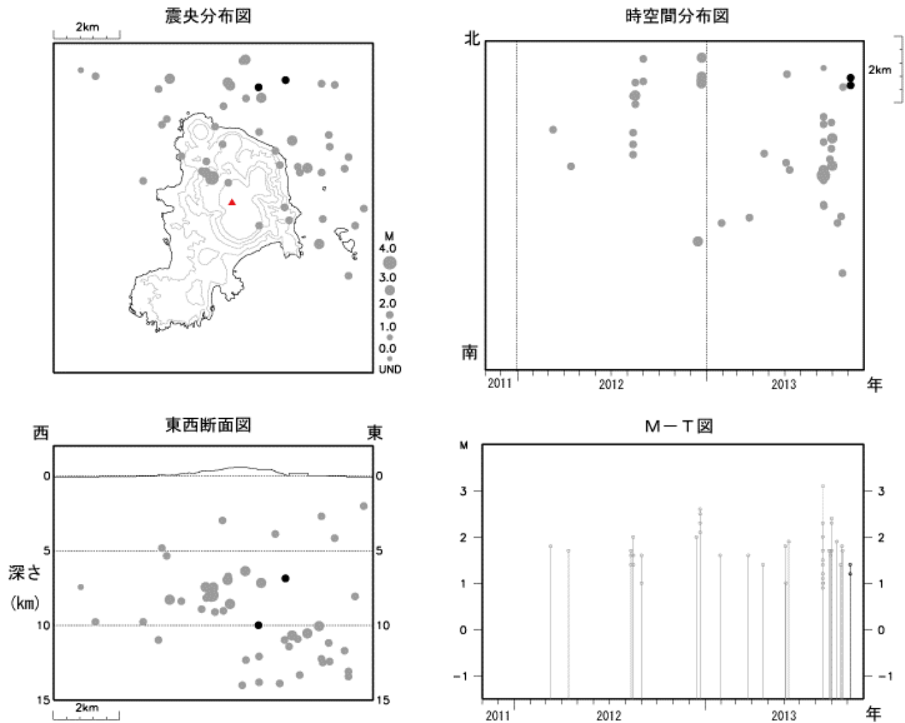
図 4 神津島 広域地震観測網による山体・周辺の地震活動（2011 年 11 月 1 日～2013 年 10 月 31 日）
