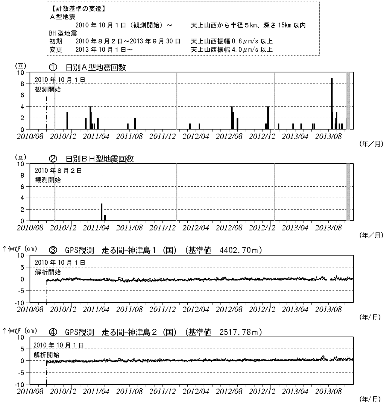
図 3 神津島 火山活動経過図(2010 年 8 月 2 日～2013 年 10 月 31 日)
