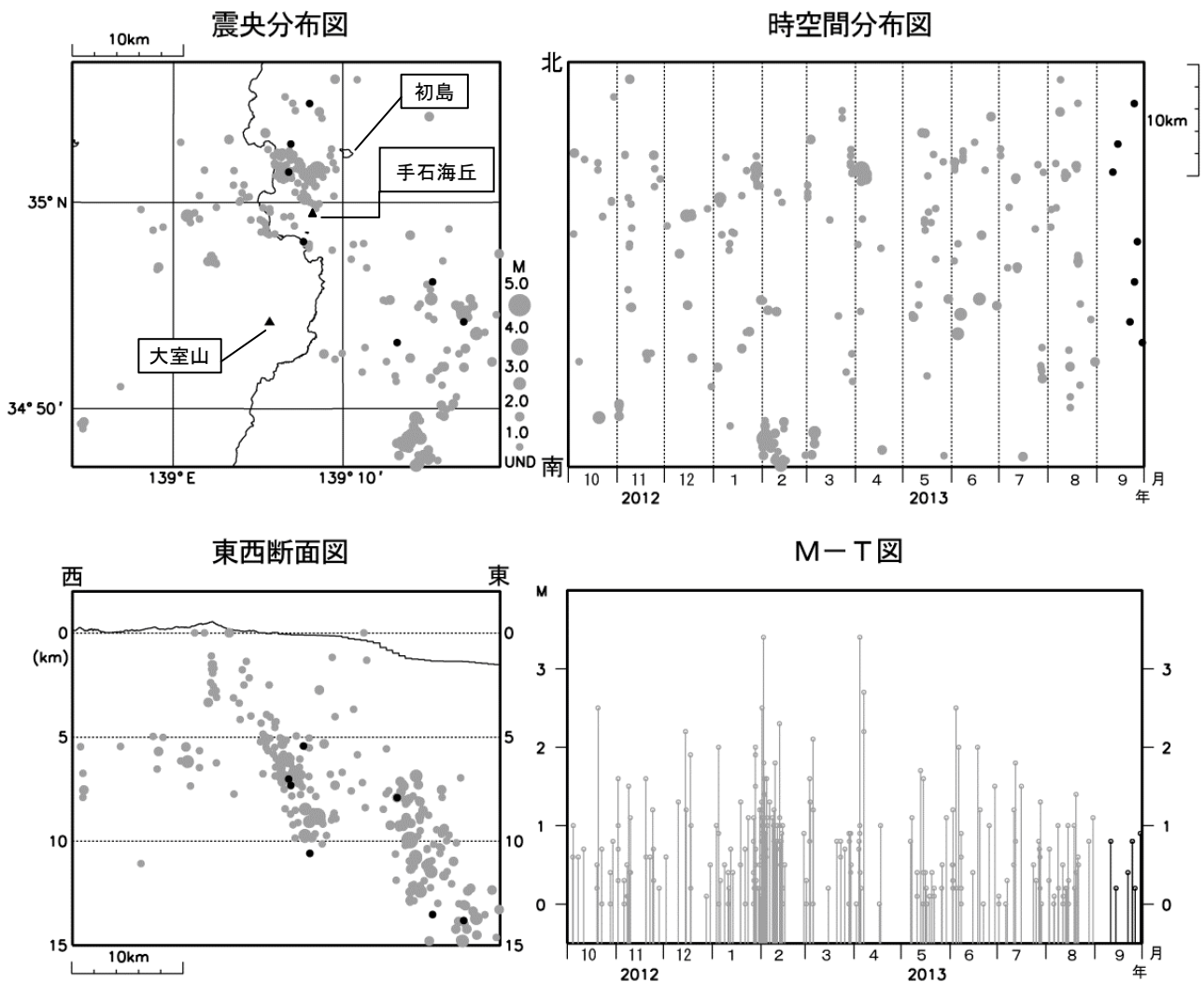
図 2 伊豆東部火山群 広域地震観測網による震源分布図（2012 年 10 月 1 日～2013 年 9 月 30 日）
