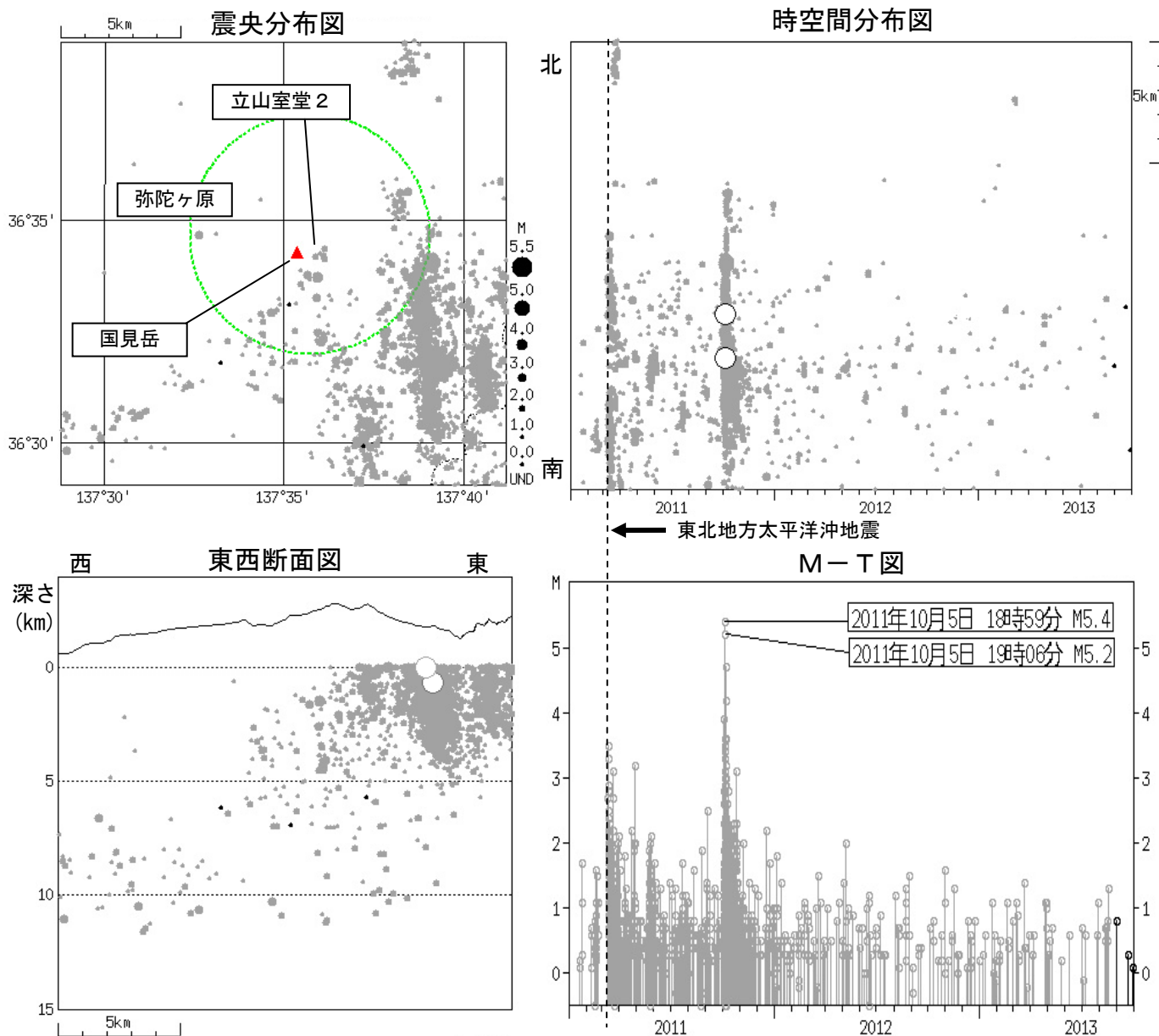
図2 弥陀ヶ原 広域地震観測網による山体・周辺の地震活動（2011年1月1日～2013年9月30日）
