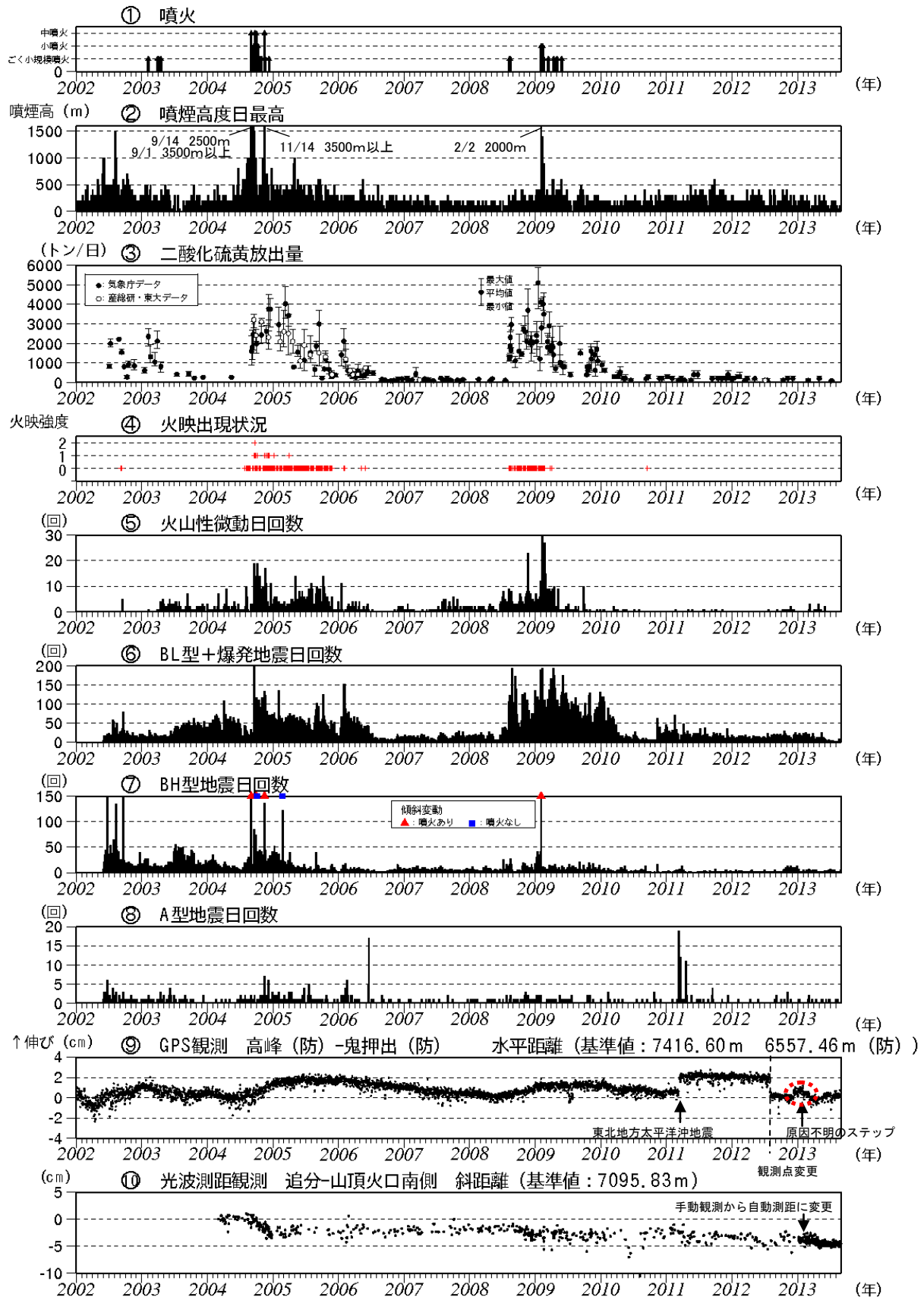
図3 浅間山 最近の火山活動経過図 (2002年1月1日～2013年8月31日)
