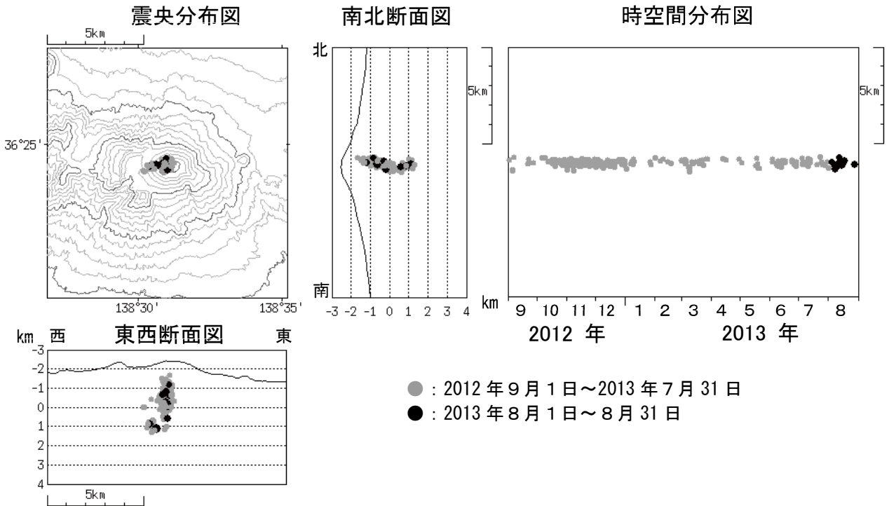
図 4 浅間山 震源分布図（2012 年 9 月 1 日～2013 年 8 月 31 日）
