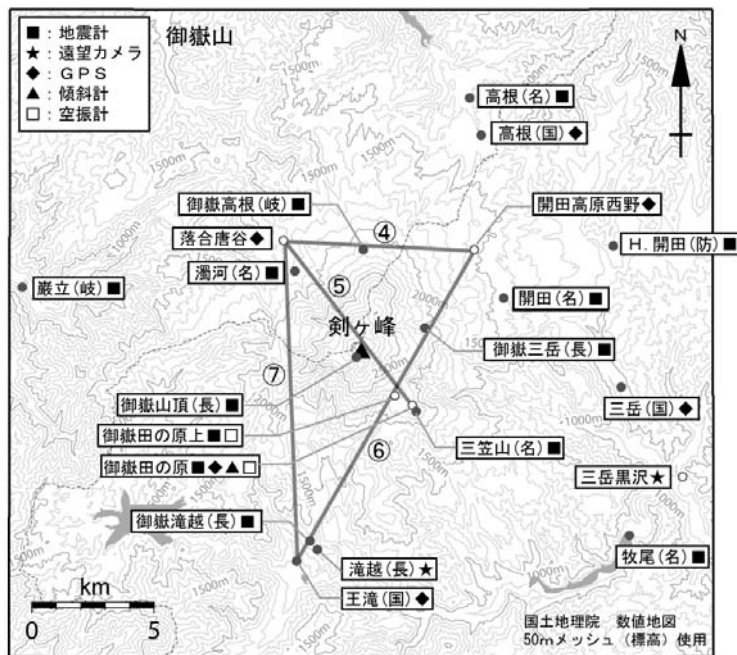
図5 御嶽山 観測点配置図
