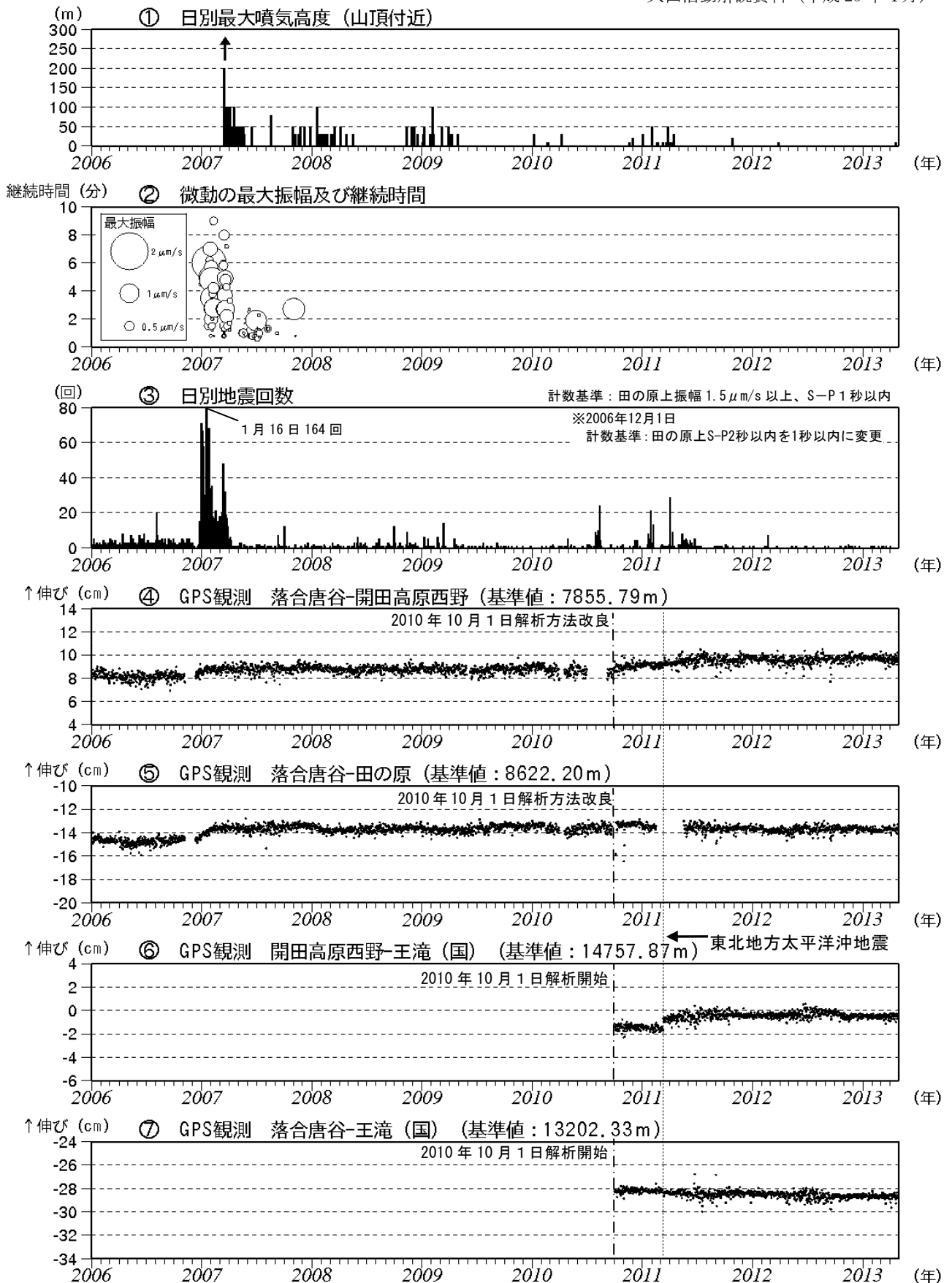
図3※ 御嶽山 最近の火山活動経過図（2006年1月1日～2013年4月30日）
