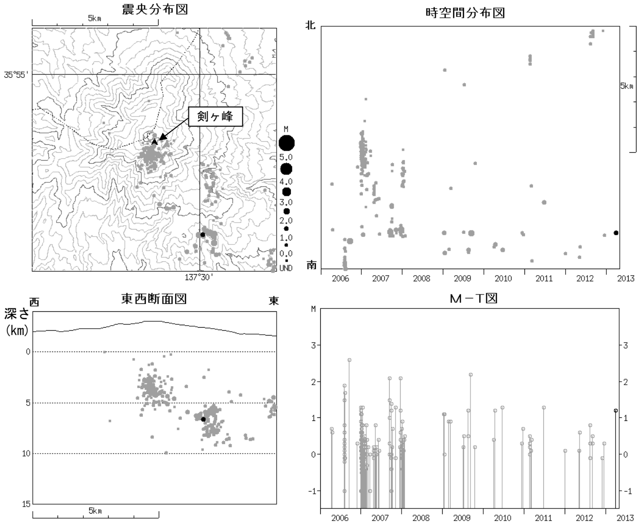
図4※ 御嶽山 広域地震観測網による山体・周辺の震源分布図（2006年1月1日～2013年4月30日）
