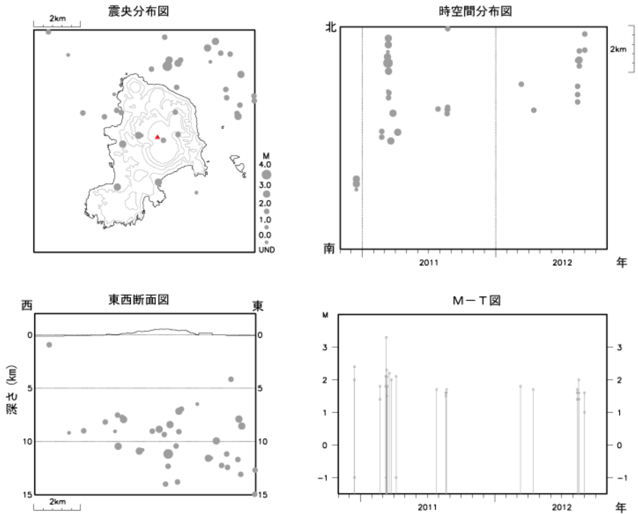
図 4 ※ 神津島 広域地震観測網による山体・周辺の地震活動（2010 年 11 月 1 日～2012 年 10 月 31 日）
