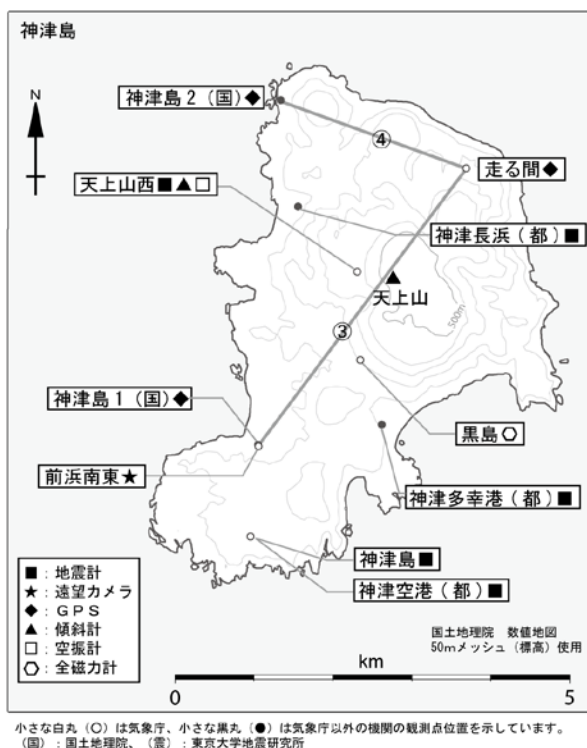
図 1 神津島 観測点配置図
