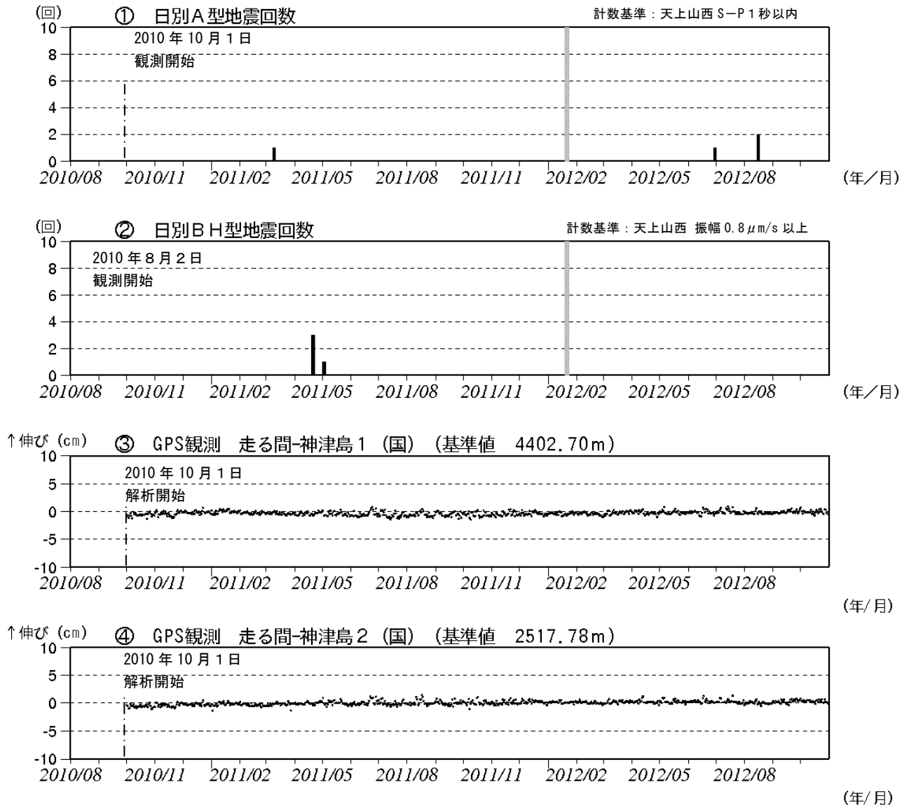
図 3 神津島 火山活動経過図(2010 年 8 月 2 日~2012 年 10 月 31 日)
