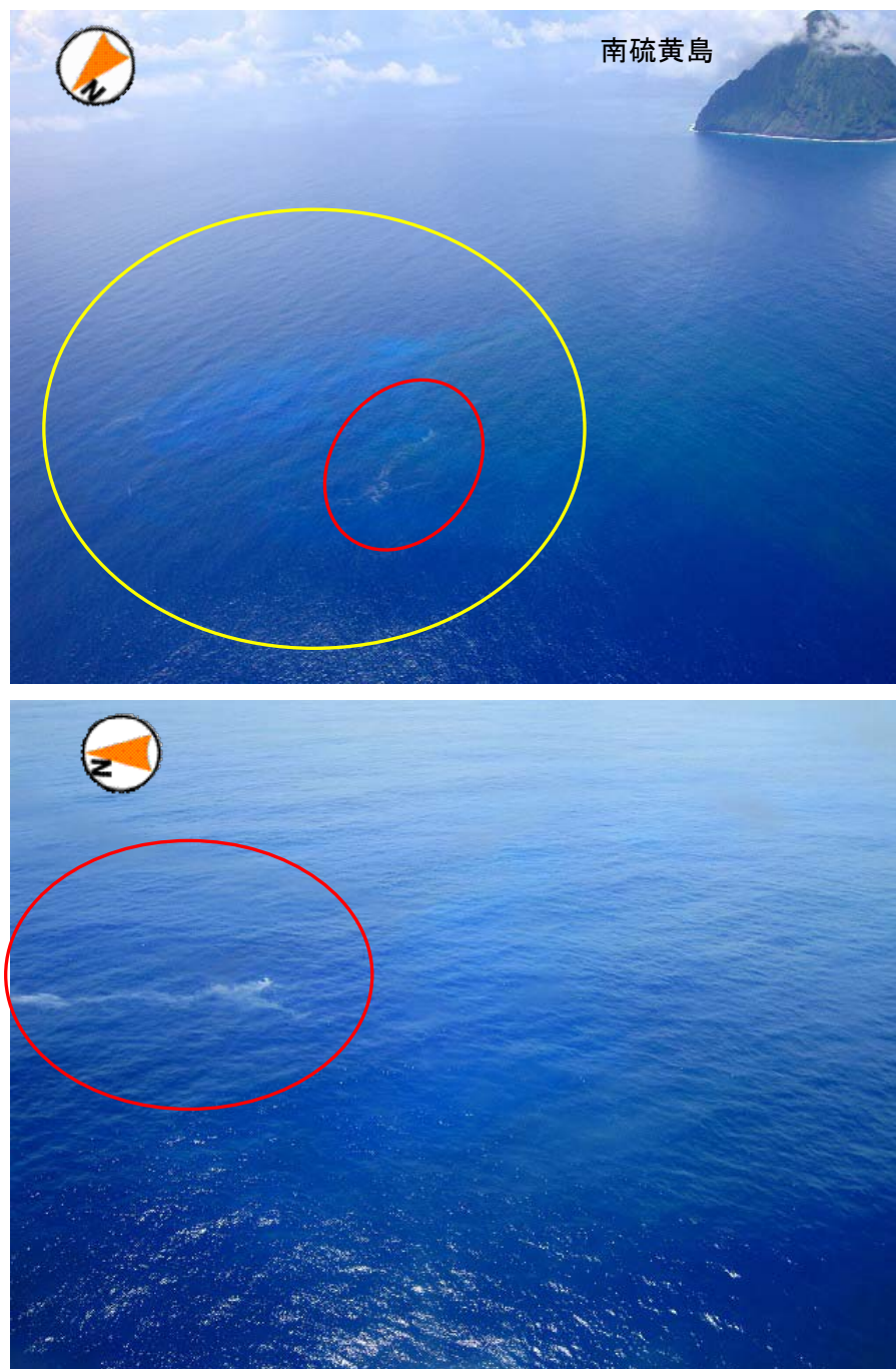
図 2 福德岡ノ場 変色水の状況 9 日 10 時 50 分頃撮影（海上自衛隊の協力による） 湧出点付近において、幅 200m、長さ 300m の青白色の変色水（黄線枠）を確認しました。 ・上図：南硫黄島の北西方向から撮影。 ・下図：上図の赤線枠付近を西方向から近接撮影。
