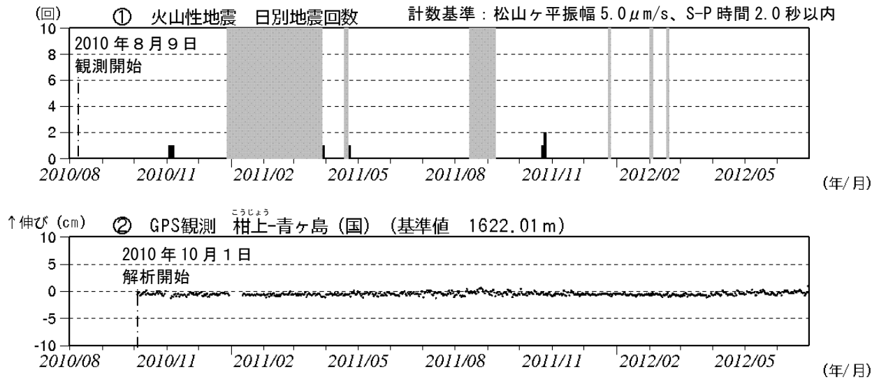
図 2 青ヶ島 火山活動の推移（2010 年 8 月 9 日～2012 年 6 月 30 日）
