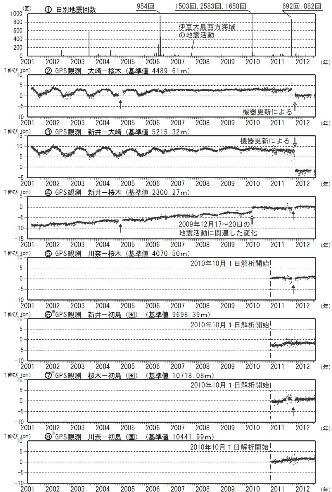
図3 伊豆東部火山群 最近の火山活動経過図（2001年1月～2012年6月）
