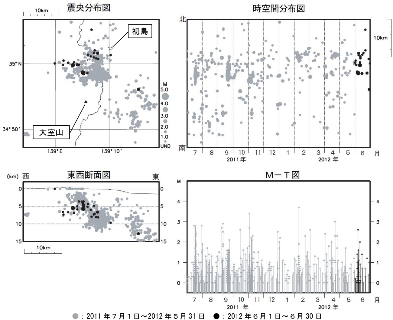
図 2 ※ 伊豆東部火山群 広域地震観測網による震源分布図（2011 年 7 月 1 日～2012 年 6 月 30 日） M（マグニチュード）は地震の規模を表します。 図中の震源要素は一部暫定値が含まれており、後日変更することがあります。
